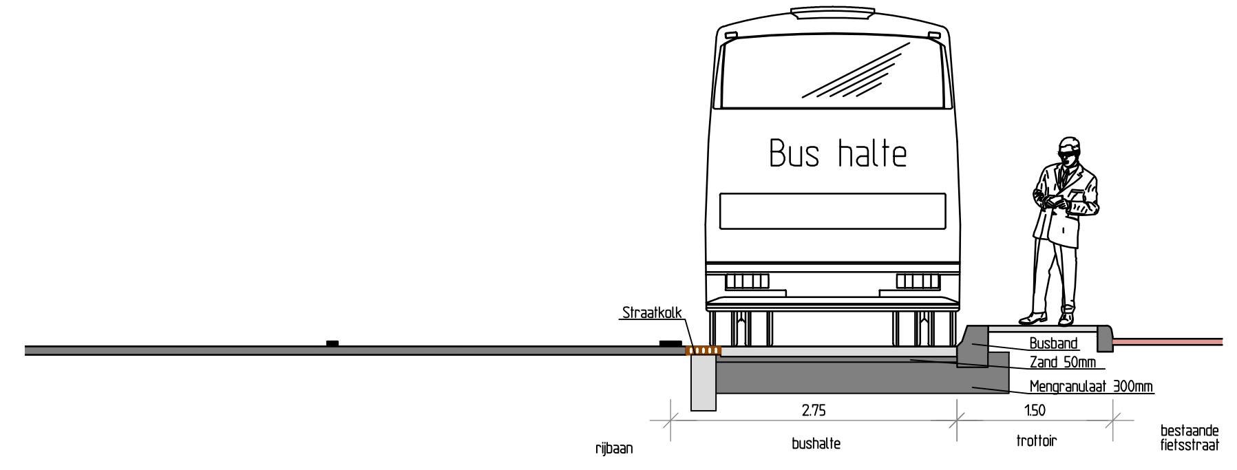
Dwarsdoorsnedes schaal 1:50
