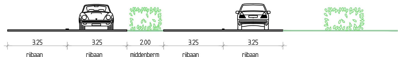
Dwarsprofiel 5
