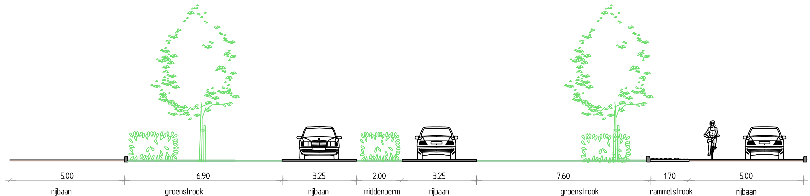
Dwarsprofiel 3
