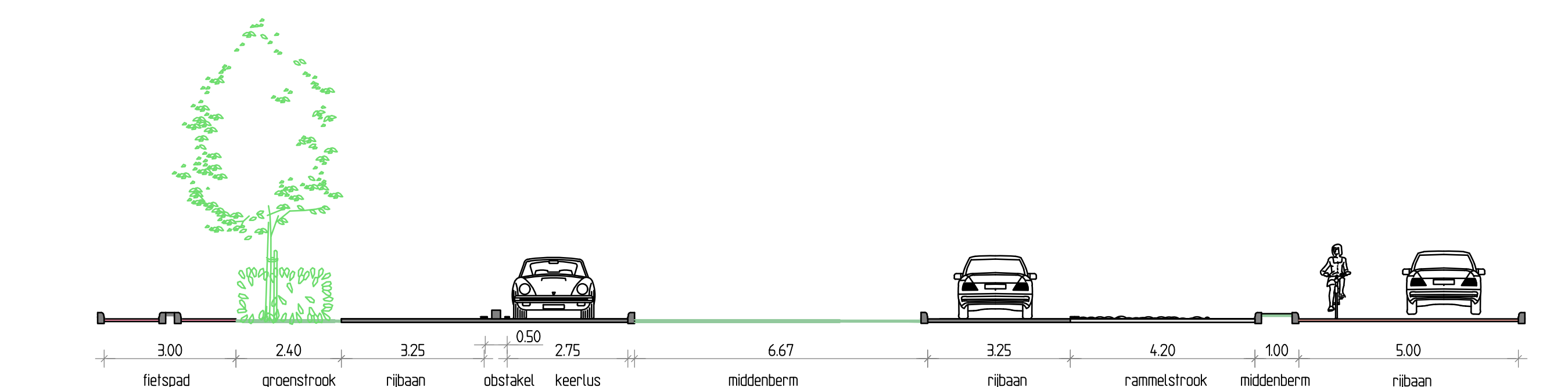
Dwarsprofiel 2
