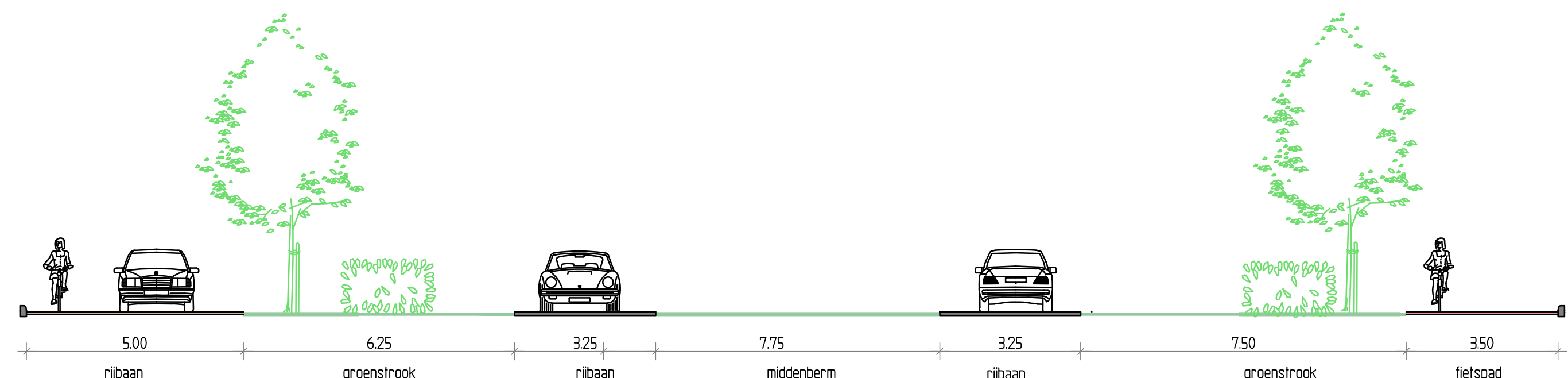
Dwarsprofiel 4
