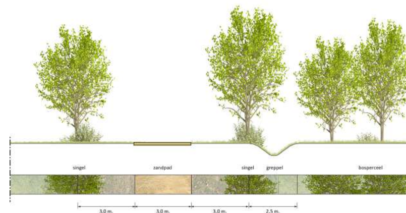
Profiel F-F' - zandpad
