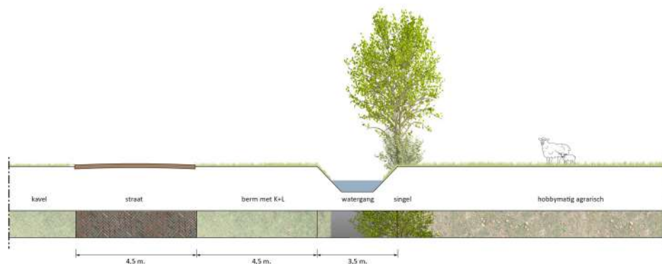
Profiel B-B' - westelijke deel noordelijke weg
