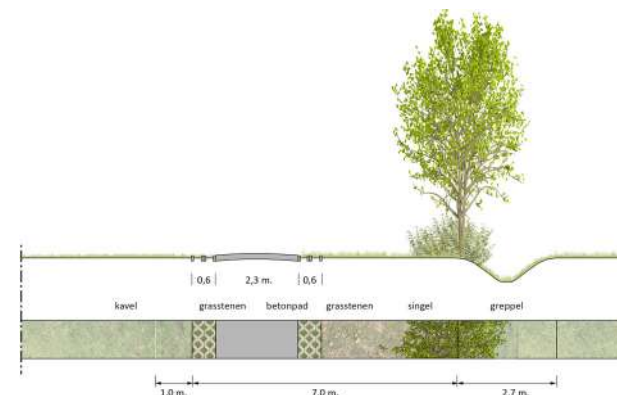
Profiel D-D' - betonpad
