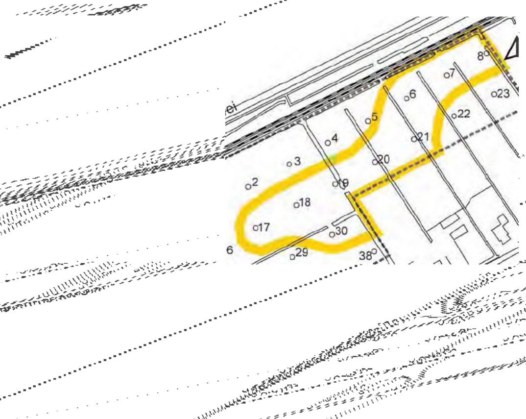
Figuur 5. Feanwâlden, 't Landeke. Boorpuntenkaart. De genummerde punten geven de uitgevoerde boringen weer. Binnen de oranje omlijnde zone is karterend booronderzoek uitgevoerd. [Bron: klic.]
