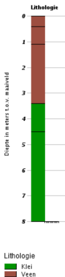
Figuur 3: Uitsnede van boring B31A0036 en B31A1183 (bron: Dinoloket.nl) .
