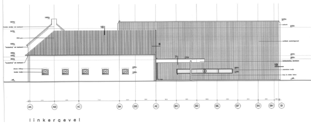
Figuur 5: gevelaanzichten
