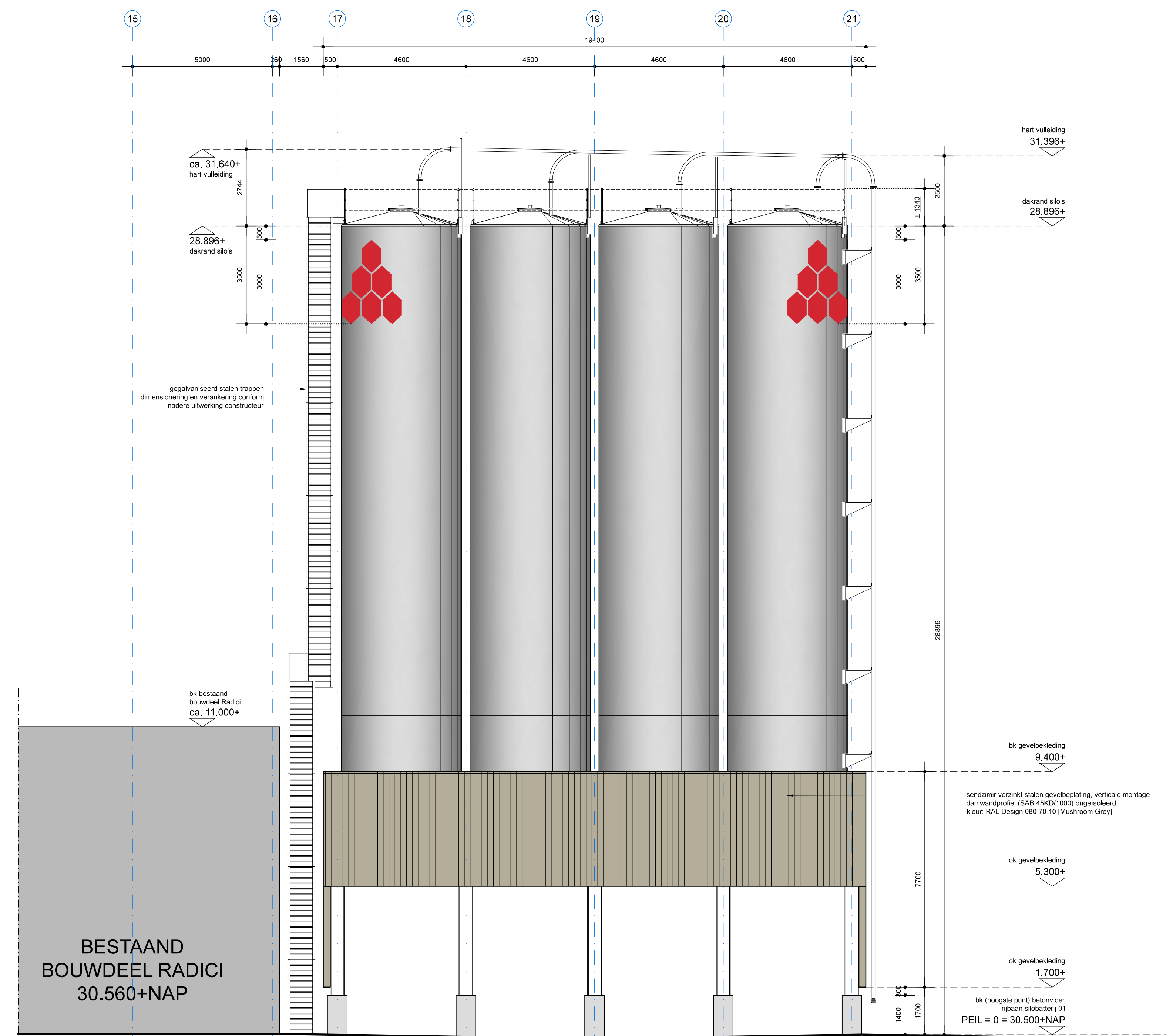
Contour rechter zijgevel bestaand bouwdeel Radici
