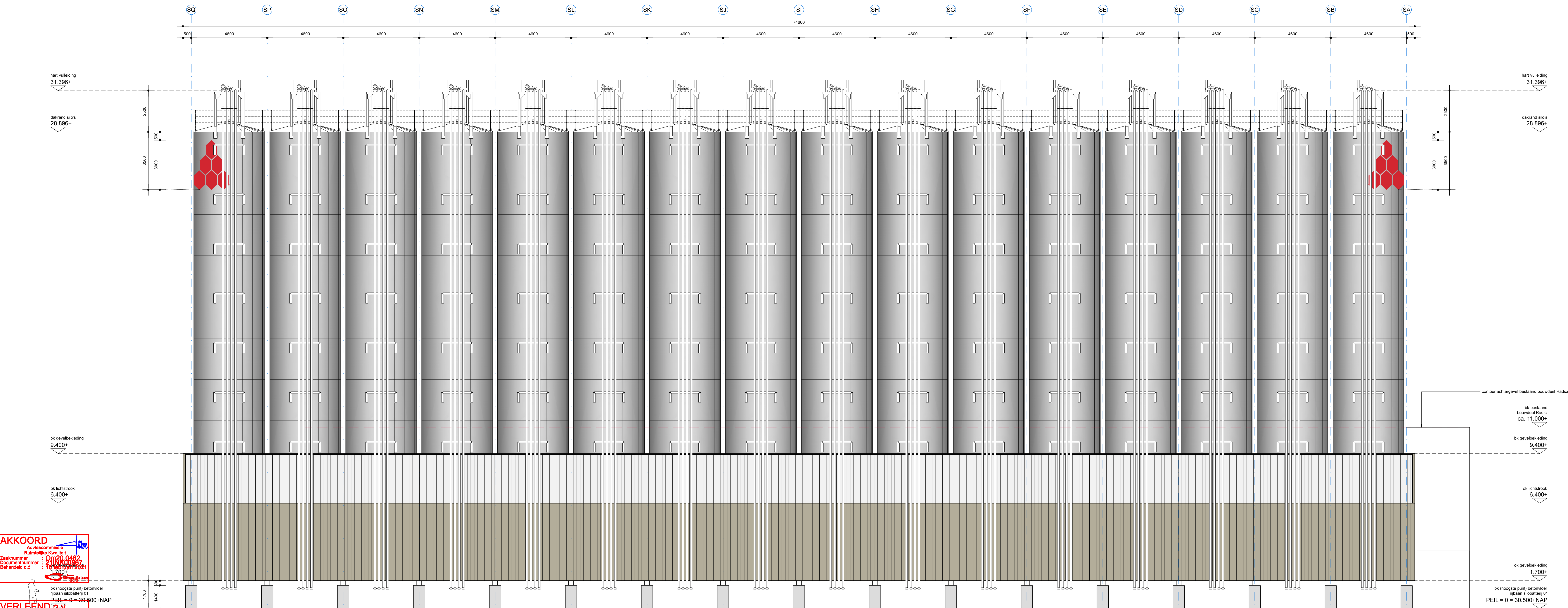
Langsgevel silobatterij 01, gevel op as 21
