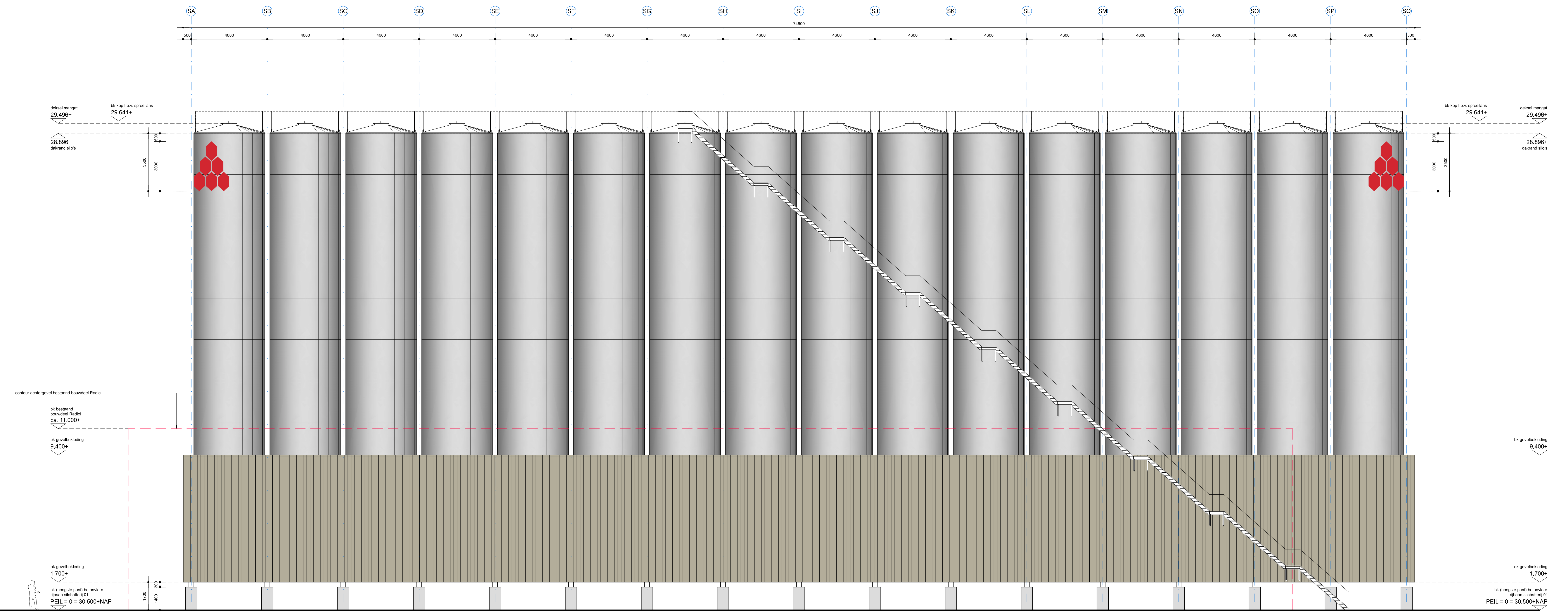
Langsgevel silobatterij 01 Tussengevel op as 17 zonder lichtstrook
