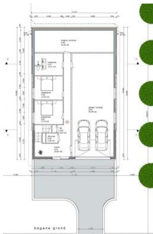
Figuur 6 bouwplan woonhuis Henssen
