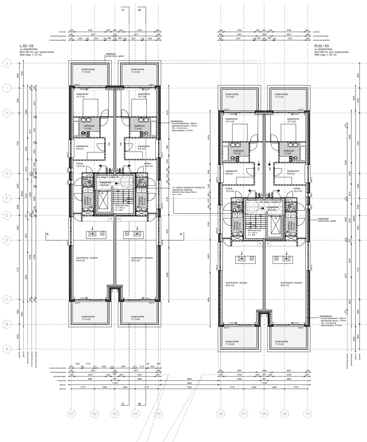
Plattegrond eerste verdieping.
