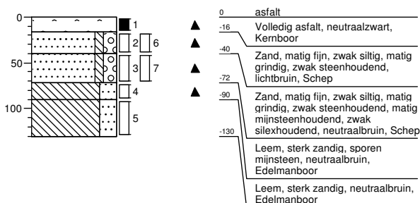
Boring: 127 Datum: 16-01-2017
