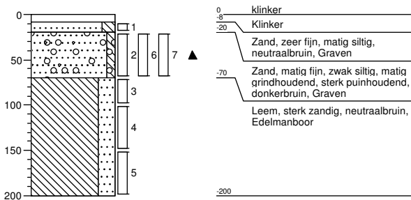
Boring: 153 Datum: 17-01-2017
