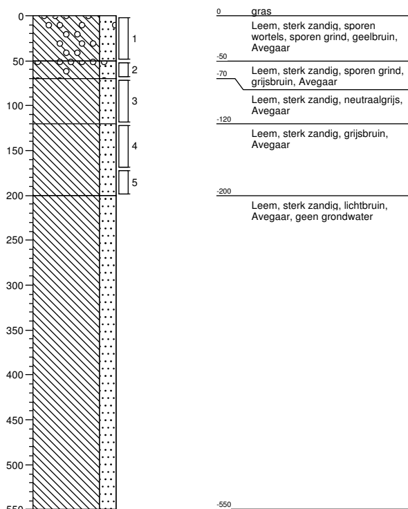
Boring: 137 Datum: 16-01-2017
