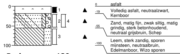
Boring: 120 Datum: 16-01-2017
