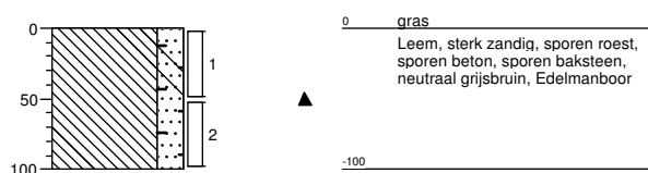
Boring: 060 Datum: 12-01-2017
