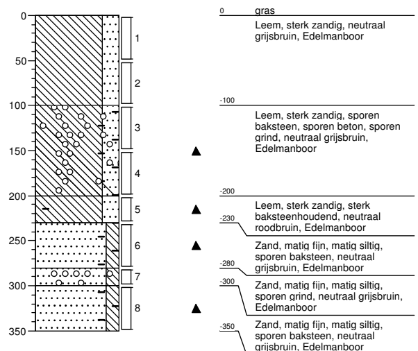
Boring: 301 Datum: 13-01-2017
