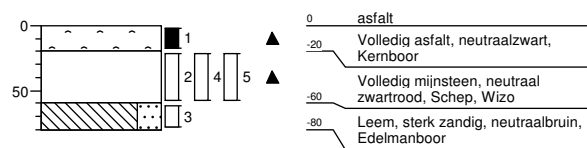
Boring: 124 Datum: 16-01-2017
