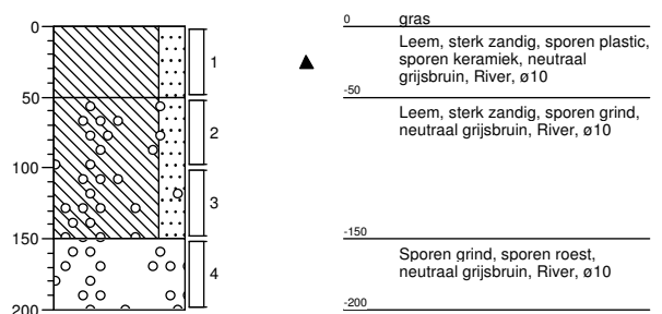
Boring: 128 Datum: 16-01-2017
