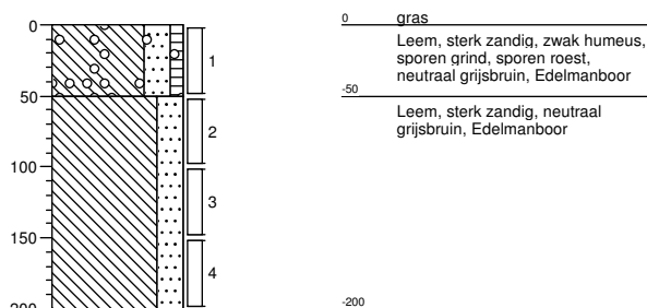
Boring: 059 Datum: 12-01-2017
