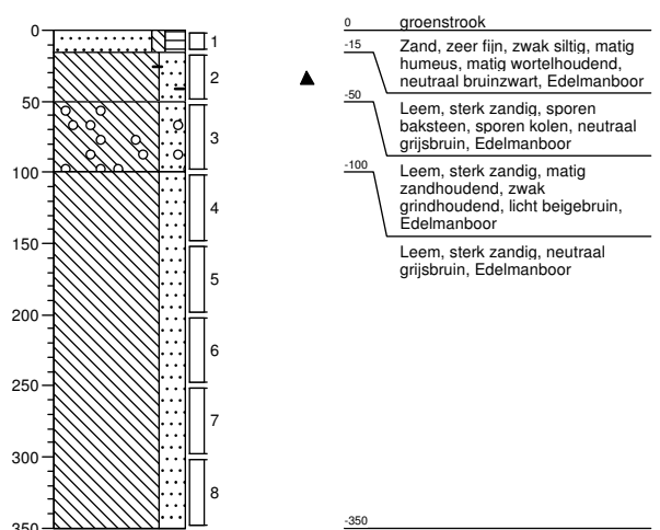
Boring: 307 Datum: 12-01-2017
