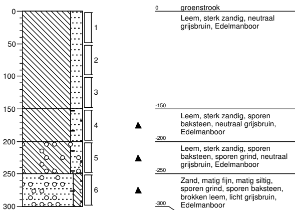
Boring: 204 Datum: 12-01-2017
