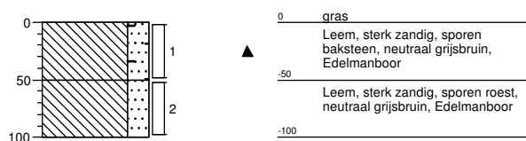
Boring: 061 Datum: 12-01-2017
