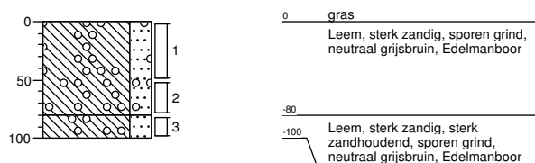
Boring: 059 Datum: 12-01-2017
