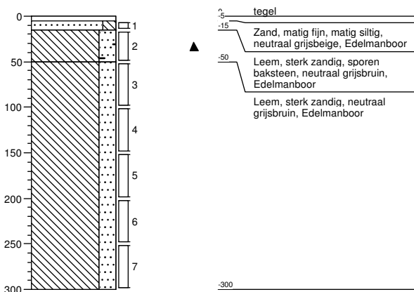
Boring: 204 Datum: 12-01-2017
