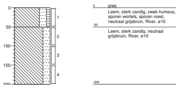
Boring: 140 Datum: 19-01-2017
