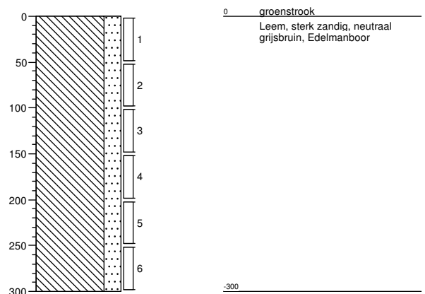
Boring: 301 Datum: 13-01-2017
