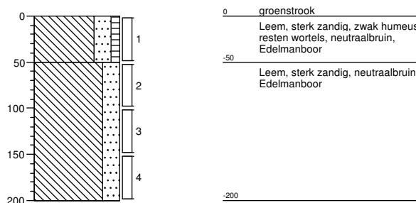
Boring: 020 Datum: 19-01-2017
