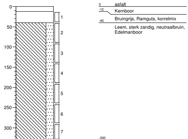
Boring: 203 Datum: 12-01-2017
