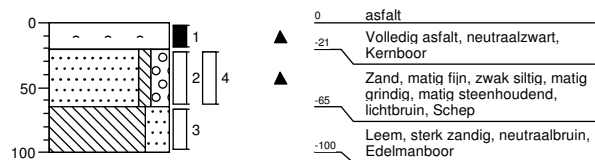
Boring: 124 Datum: 16-01-2017
