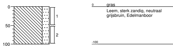
Boring: 001 Datum: 13-01-2017
