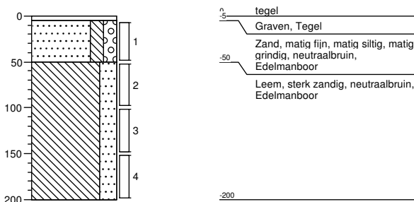
Boring: 125 Datum: 16-01-2017
