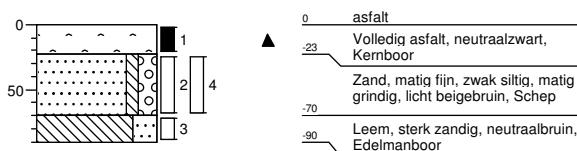
Boring: 127 Datum: 16-01-2017
