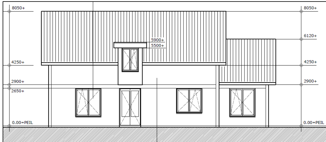
Voorgevel (oostgevel) van de nieuwe woning
