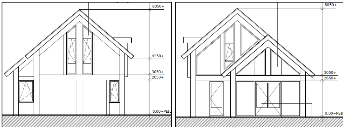
Linker zijgevel (zuidgevel) van de nieuwe woning
