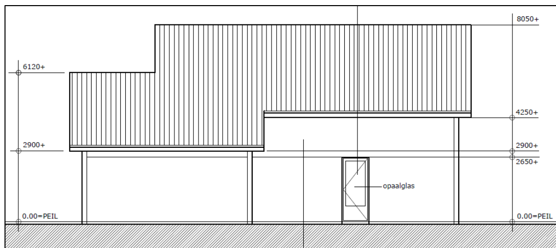
Achtergevel (westgevel) van de nieuwe woning
