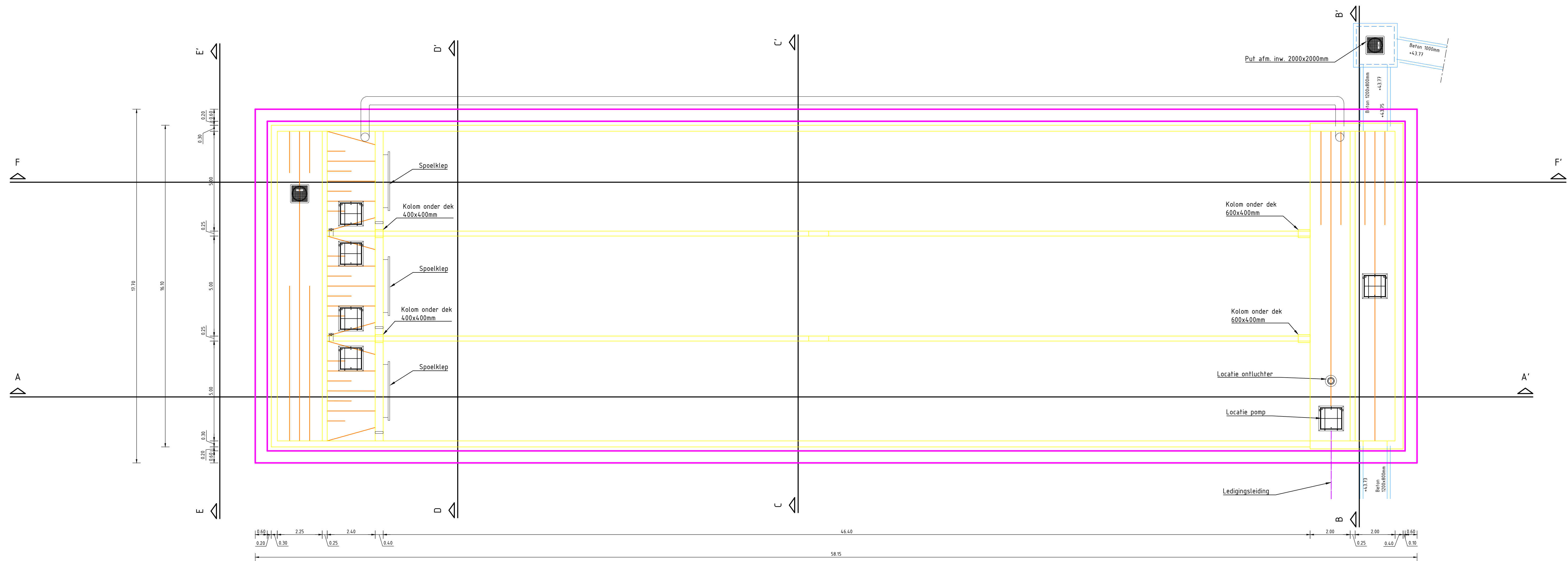
Bovenaanzicht Schaal 1:100
