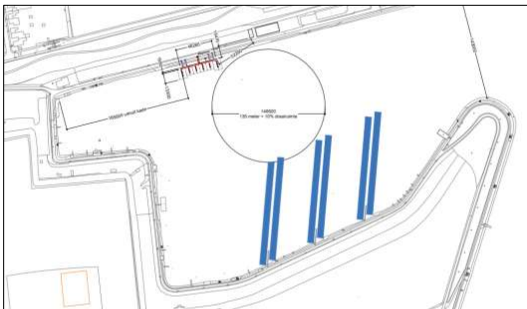
Draaicirkel beroepsvaart
