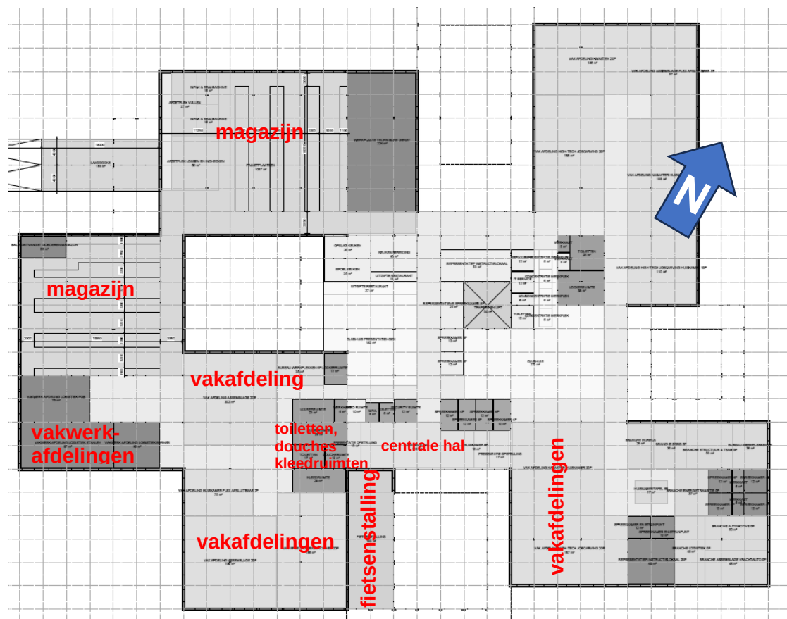
Figuur 1: Indeling gebouw ter plaatse van de zuidoost en zuidwestgevel.
