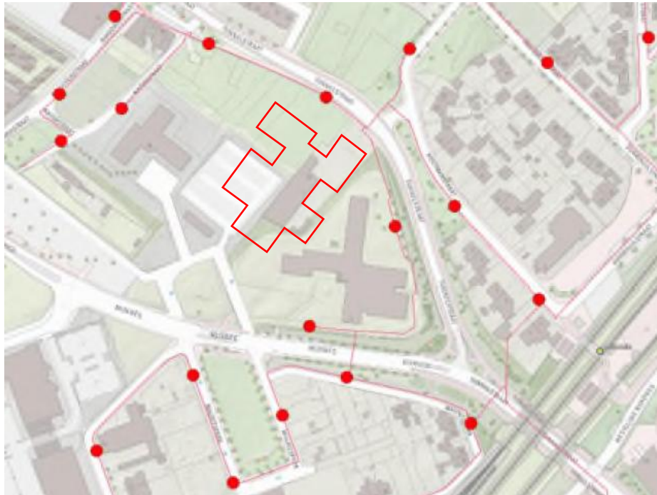
Figuur 12: aanwezigheid bluswatervoorzieningen (hydranten)
