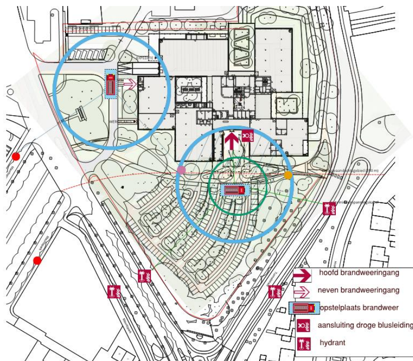
Figuur 13: brandweeringangen, aansluiting dbl en opstelplaatsen brandweer
