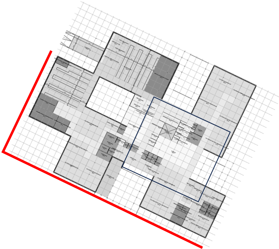
Figuur 6: gevels waar geadviseerd wordt schervvrij glas toegepast moet worden
