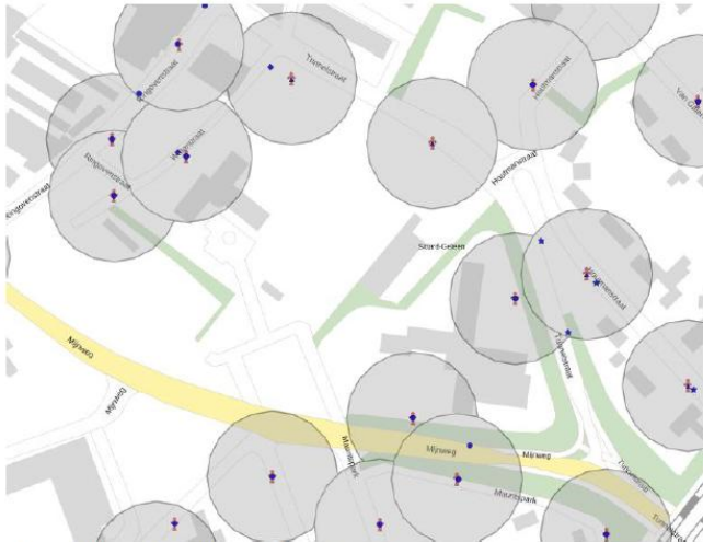
Afbeelding 4: huidige bluswatervoorzieningen
