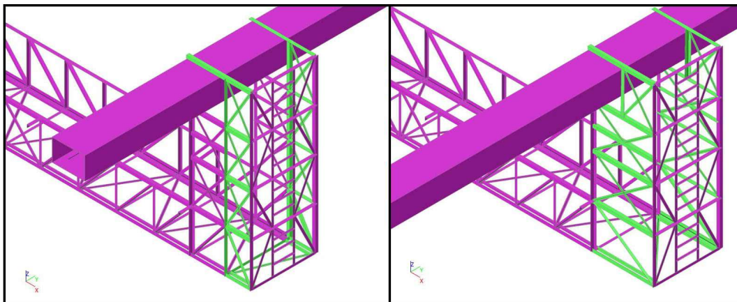
Figuur 2 – aanpassing inspectiewagen
