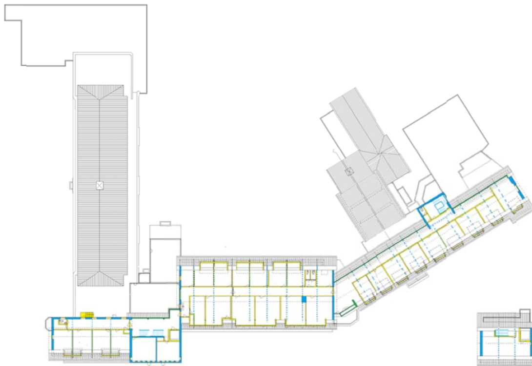
80. Monumentale waarderingsplattegrond van de zolderverdiepingen (voor groter formaat zie bijlagen)
