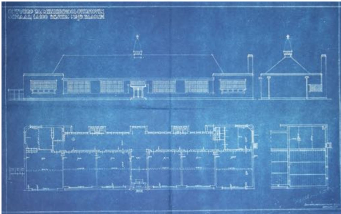
29. Ontwerptekening met plattegrond en voorgevel van de St. Jozef meisjesschool van architect Wielders uit 1925 (bron EHC, nr.995, archief architect Jos Wielders, bestek nr. 73)
