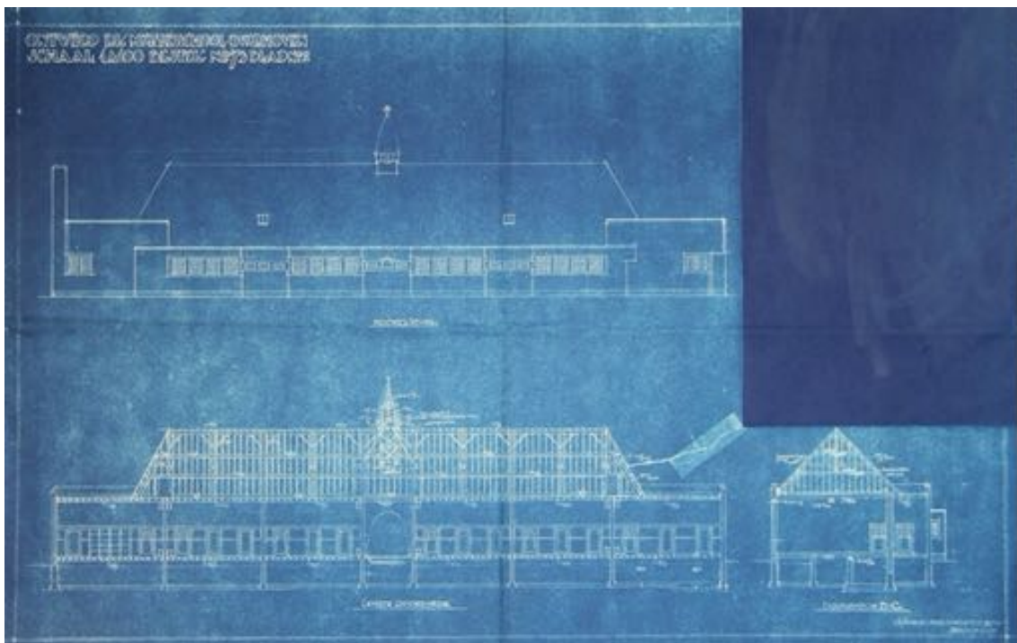
30. Ontwerptekening met doorsneden en deachtergevel van de St. Jozef Meisjesschool van architect Wielders uit 1925 (bron EHC, nr.995 archief architect Jos Wielders, bestek nr 73)
