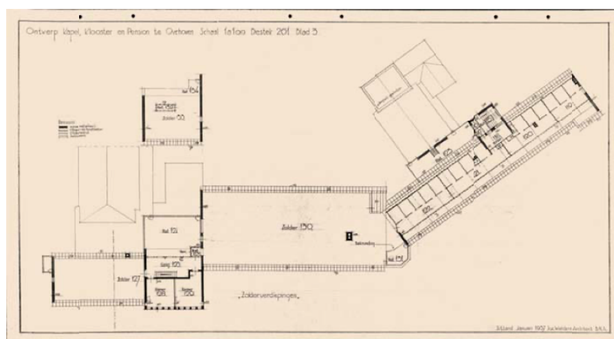
► 34. bestektekening 2 e verdieping Mariahof van architect Wielders uit 1937 (bron EHC, nr.995, archief architect Jos. Wielders, bestek nr 261)
