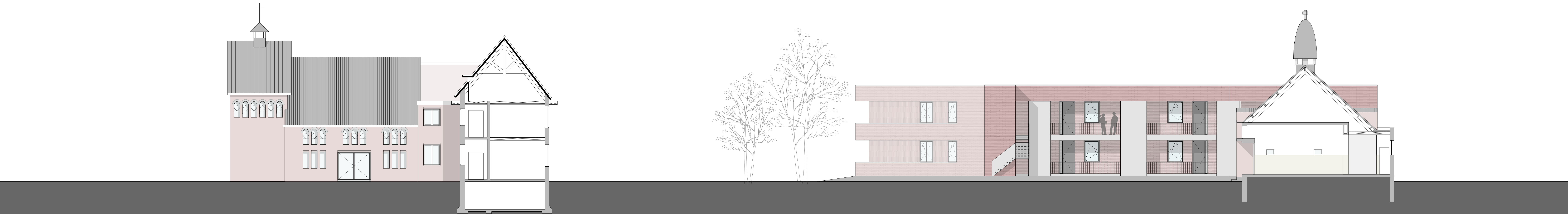
aanzicht / doorsnede G-G
