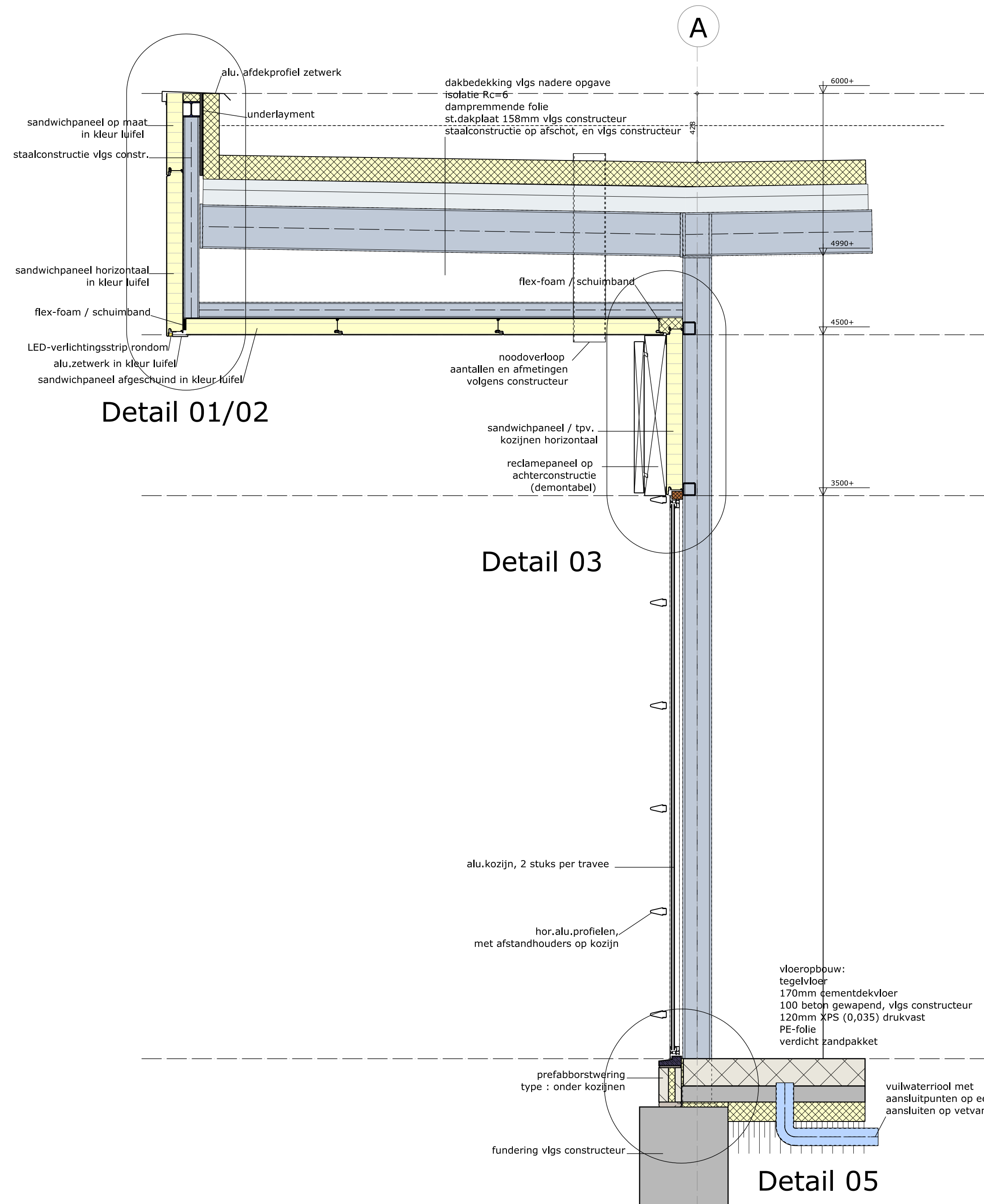
gevelprofiel P01 gevel as A en J
