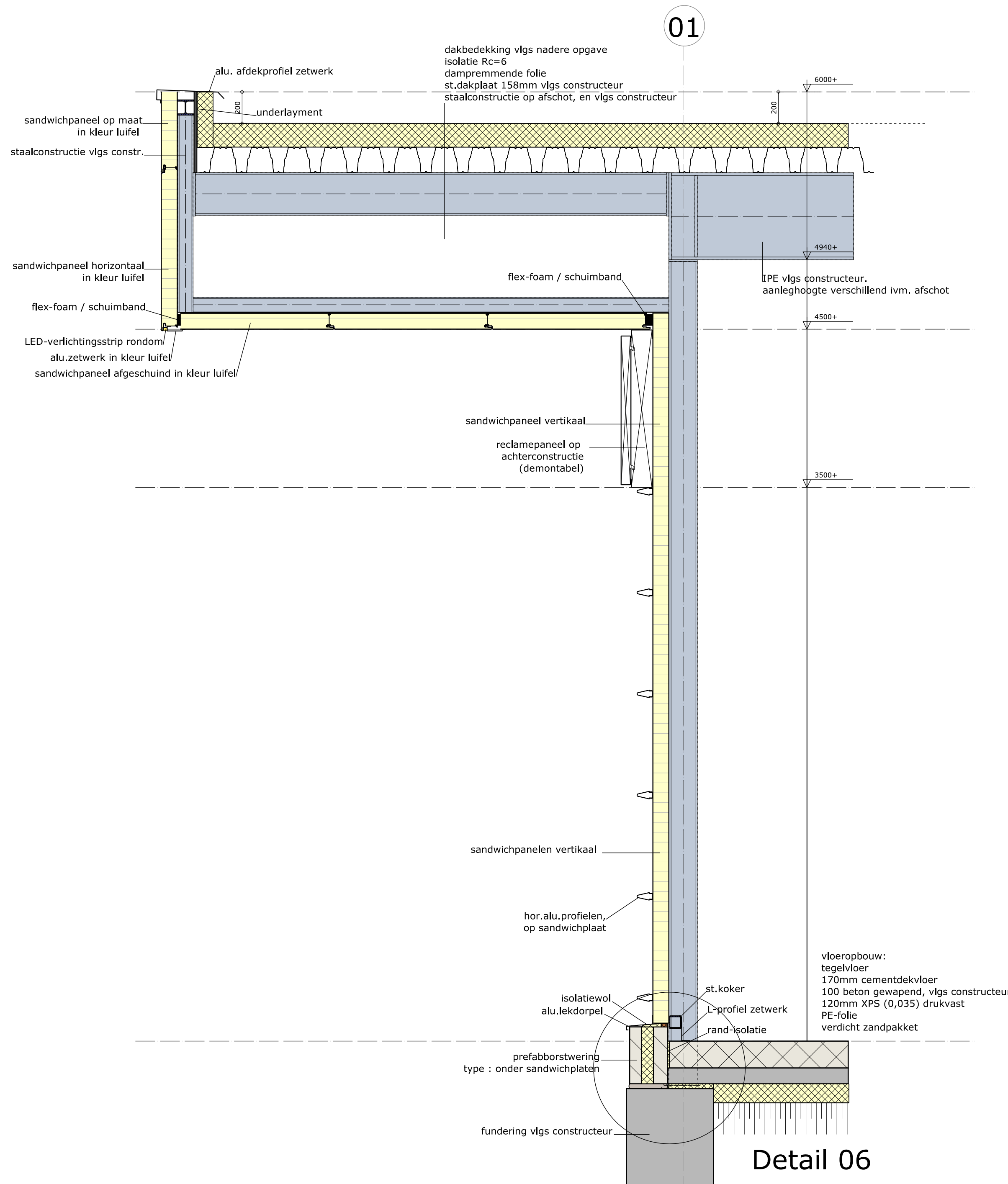
gevelprofiel P02 gevel as 1 en 12
