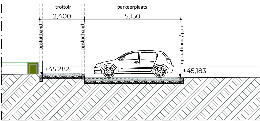
Profieldoorsnede PP
