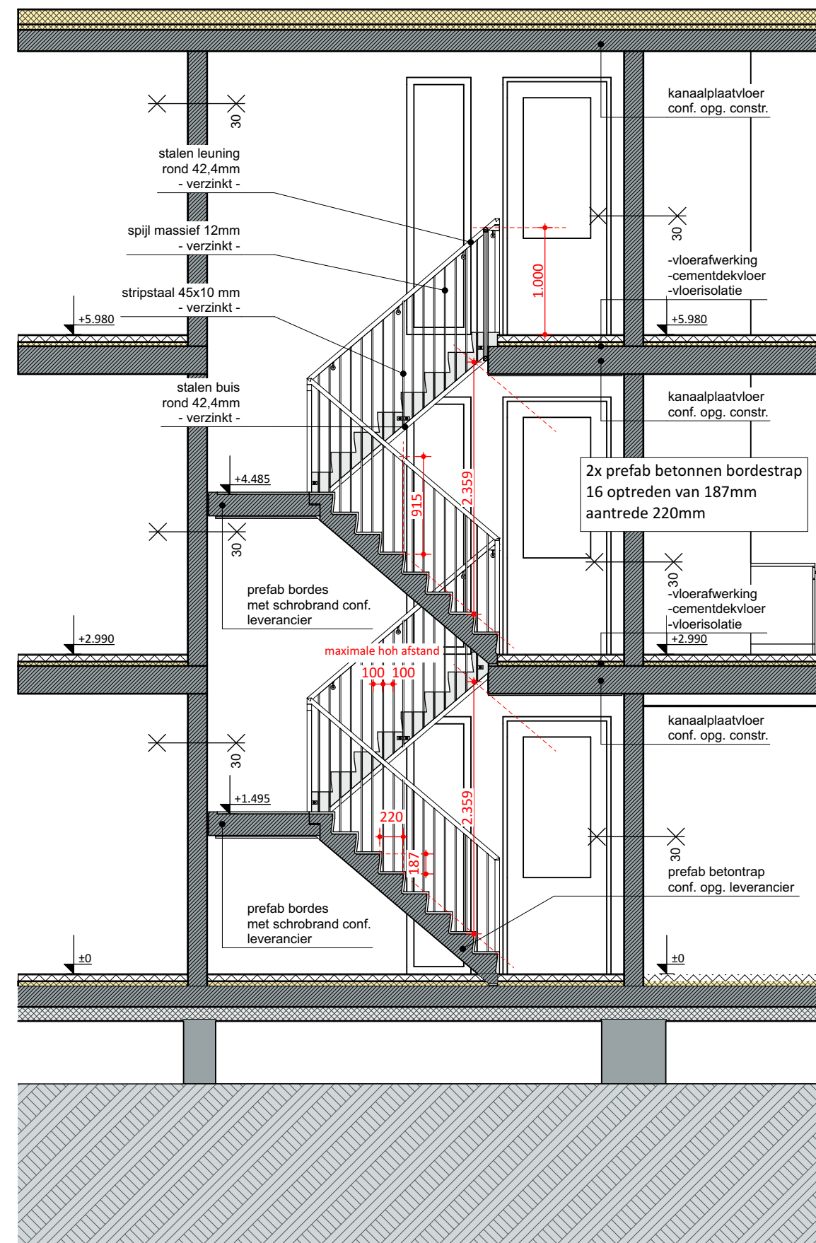
T1 Doorsnede - Trap 1:50
