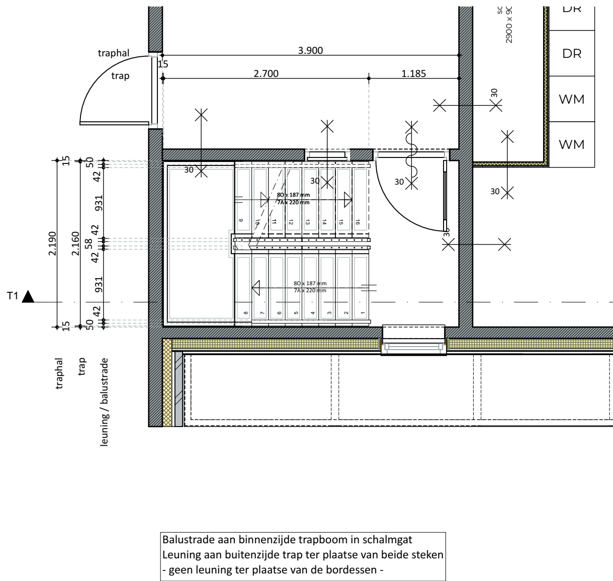
1. 1e verdieping - Trap 1:50
