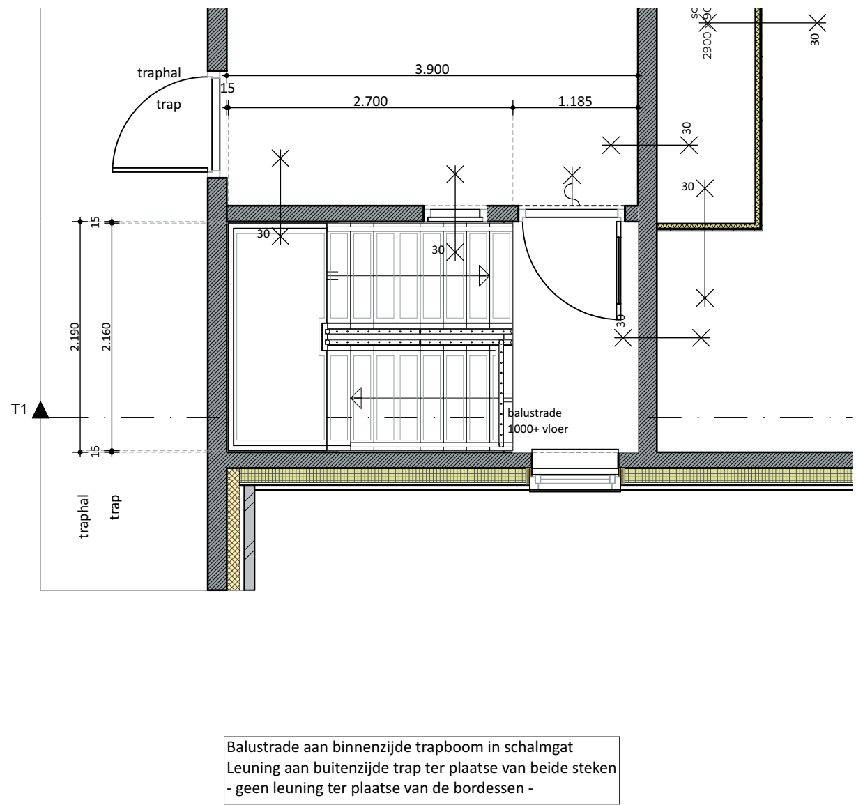
2. 2e verdieping - Trap 1:50
