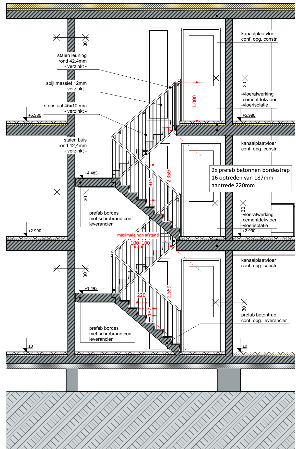
T1 Doorsnede - Trap 1:50
