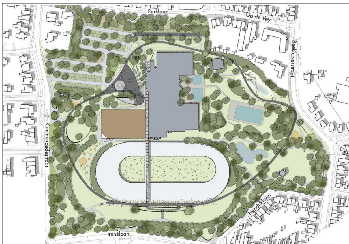
Voorlopig ontwerp (Poelmans Reesink, 2022)
