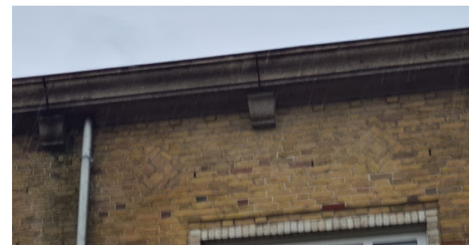
Figuur 14: Open stootvoegen onder de dakrand van Mauritspark 1A
