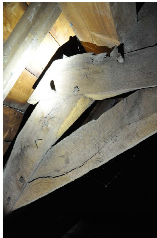
62 detail van een telmerk 'V' op een van de spanten
