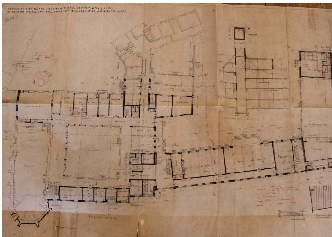
28 ontwerptekening uit 1965 van H. Palmen met in zwart alle nieuw gebouwde onderdelen op begane grond niveau.
