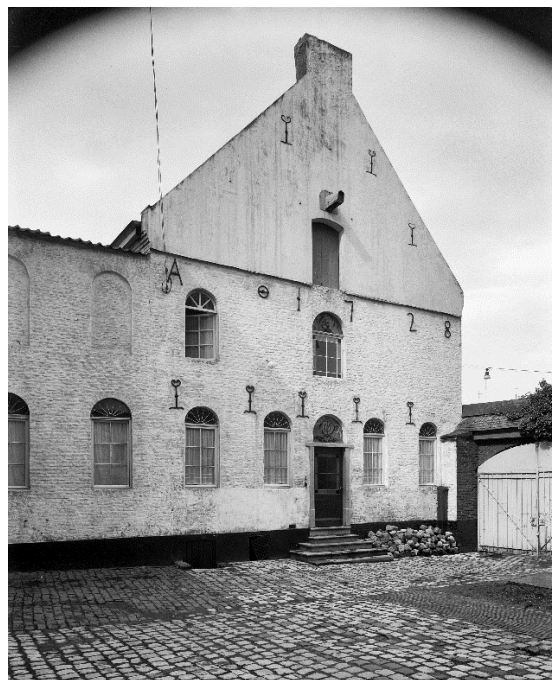
8 de zijgevel van het Jonckvrouwenhuis met jaarankers.
