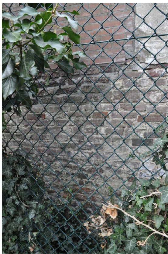
87 het oude muurwerk van handgevormde steen is opgehoogd met modern muurwerk van machinale baksteen
