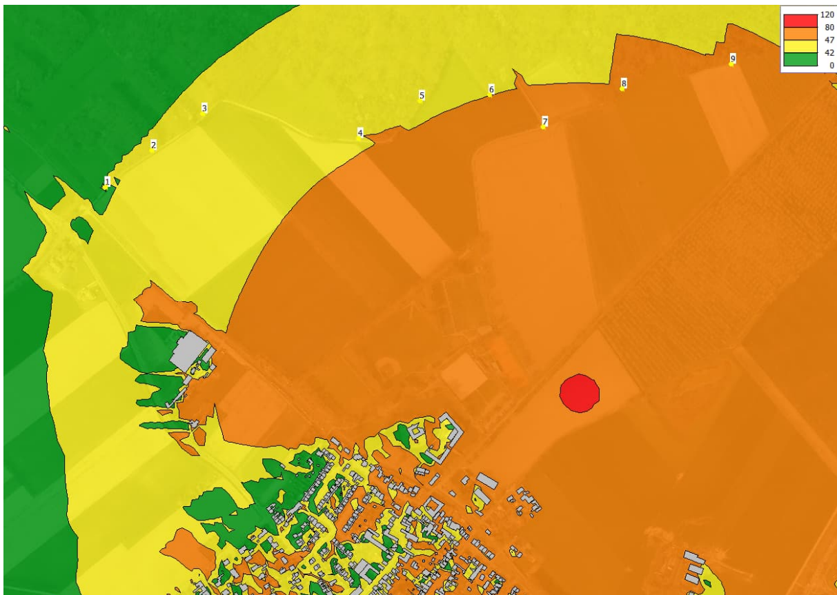
Figuur 3 - 24-uurs equivalente 42 dB(A) en 47 dB(A) geluidcontouren t.g.v. evenement in wei.
