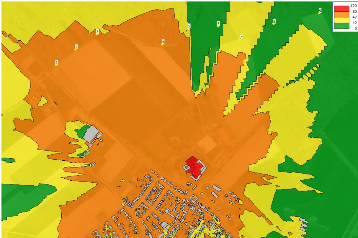
Figuur 2 - 24-uurs equivalente 42 dB(A) en 47 dB(A) geluidcontouren t.g.v. evenement bij Kasteel Limbricht.
