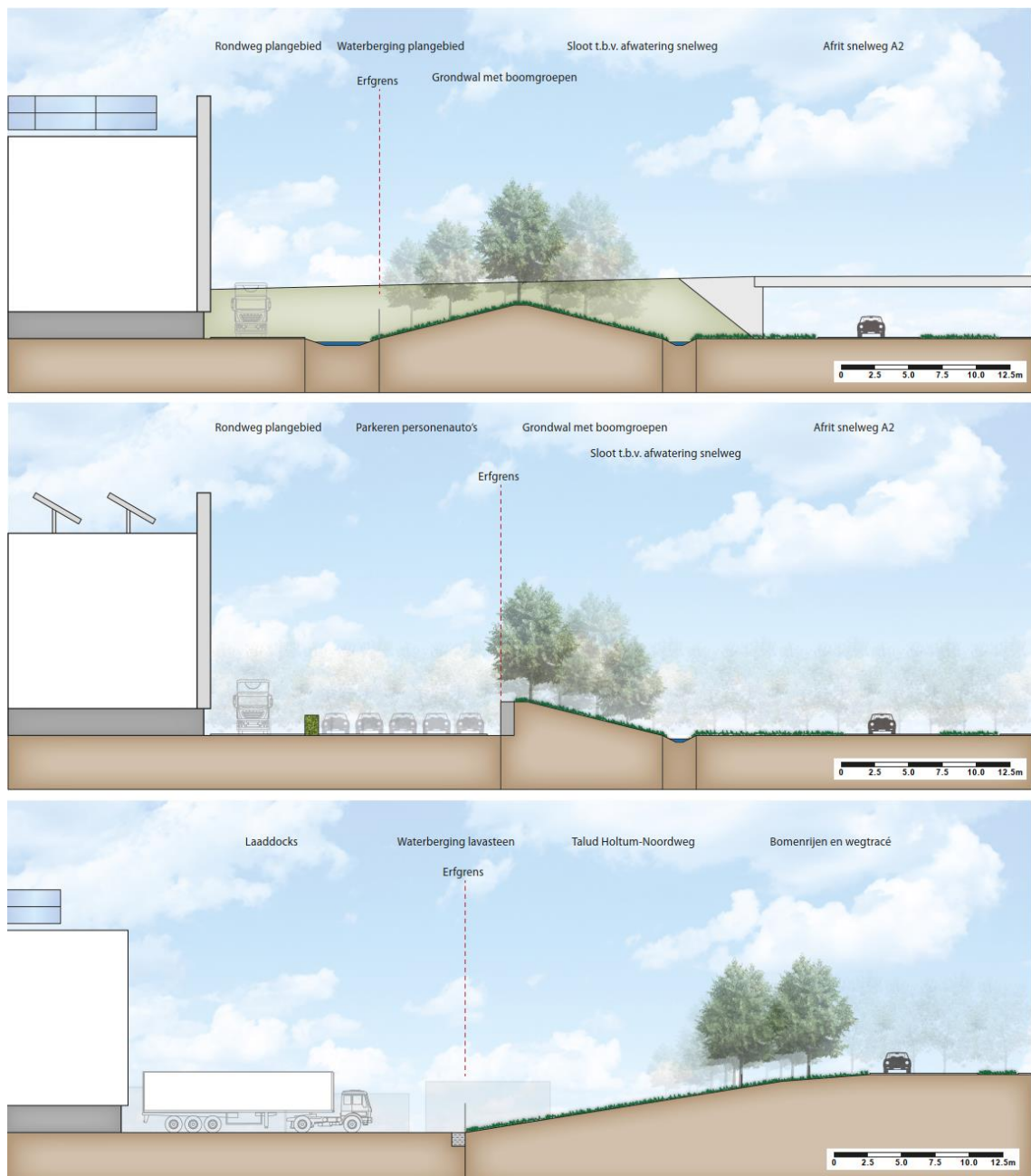
Afbeelding 5. Doorsnedes met een impressie van de toekomstige situatie.
