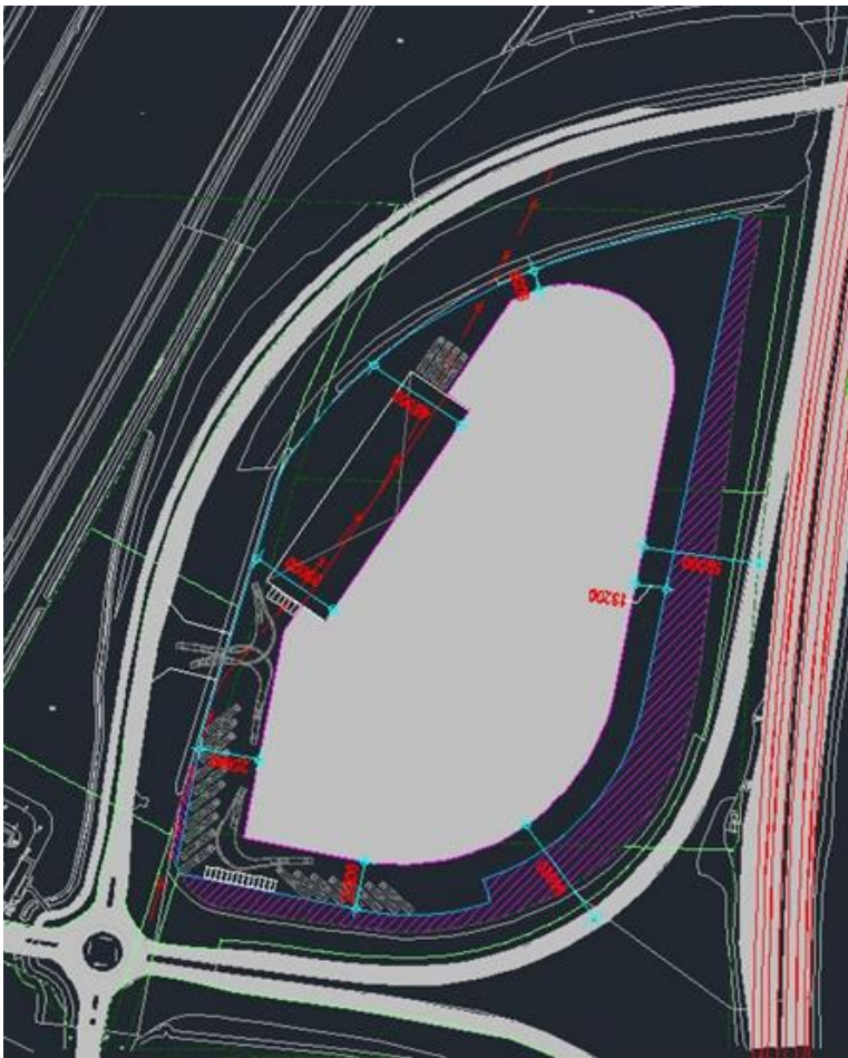
Afbeelding 4. Situatietekening, met een impressie van de toekomstige situatie.
