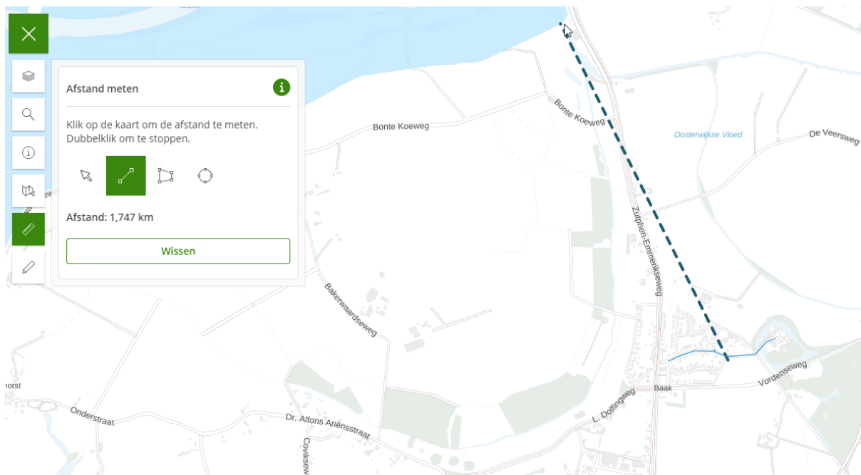
Figuur 3 - Natura 2000-gebied De Rijntakken
