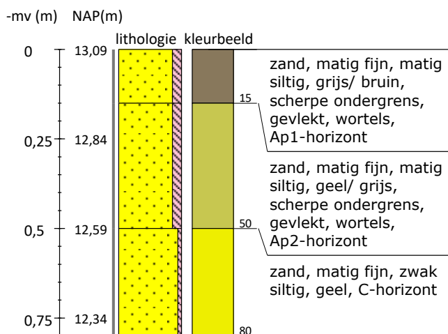
Boring 3 RD-coördinaten: 211115/446505
