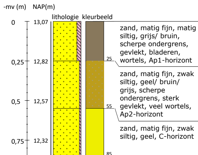
Boring 4 RD-coördinaten: 211148/466477
