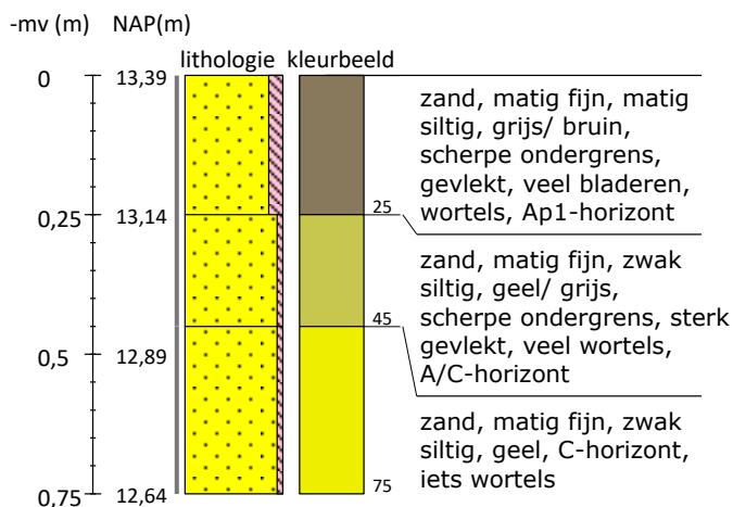
Boring 1 RD-coördinaten: 211113/446525
