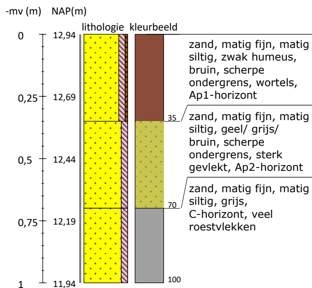
Boring 4 RD-coördinaten: 211148/466477
