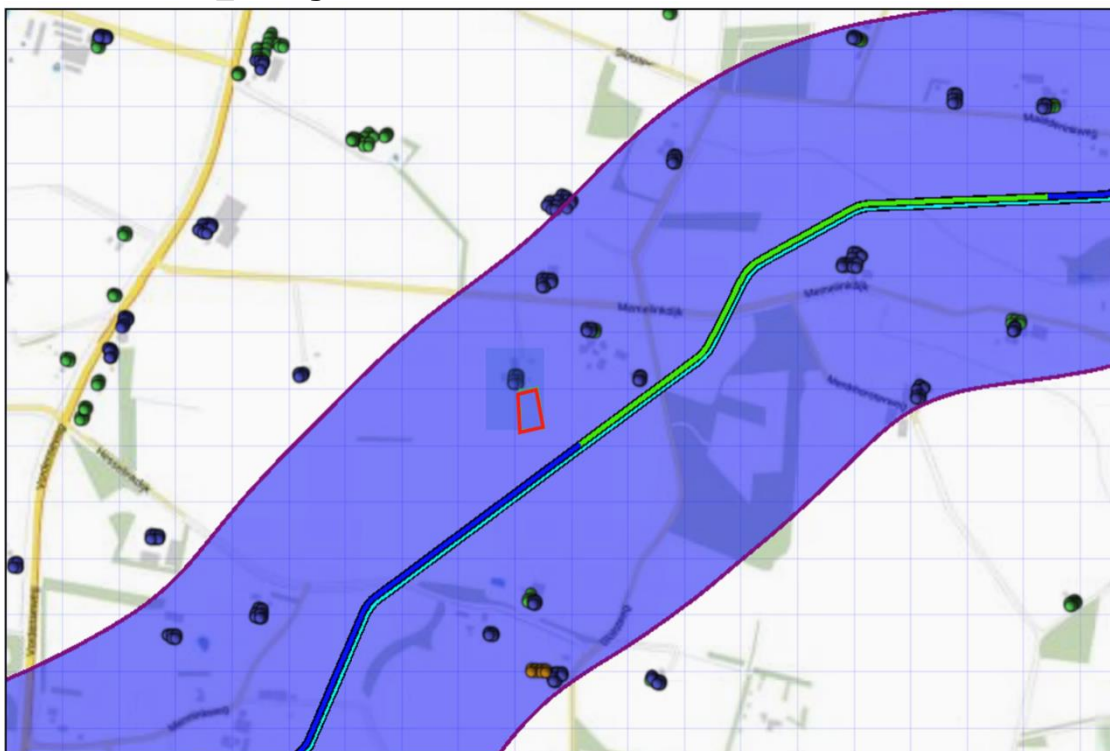
Figuur 4.2 Kilometer leiding behorende bij de maximale overschrijding van de FN-curve voor 7534_leiding-A-529-deel-1 van N.V. Nederlandse Gasunie
