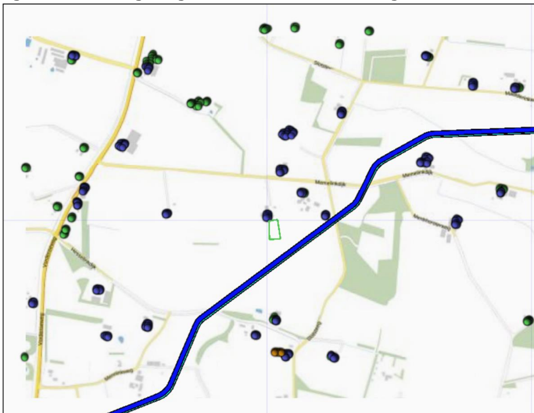
Figuur 2.3 Bevolking meegenomen in de risicoberekeningen
