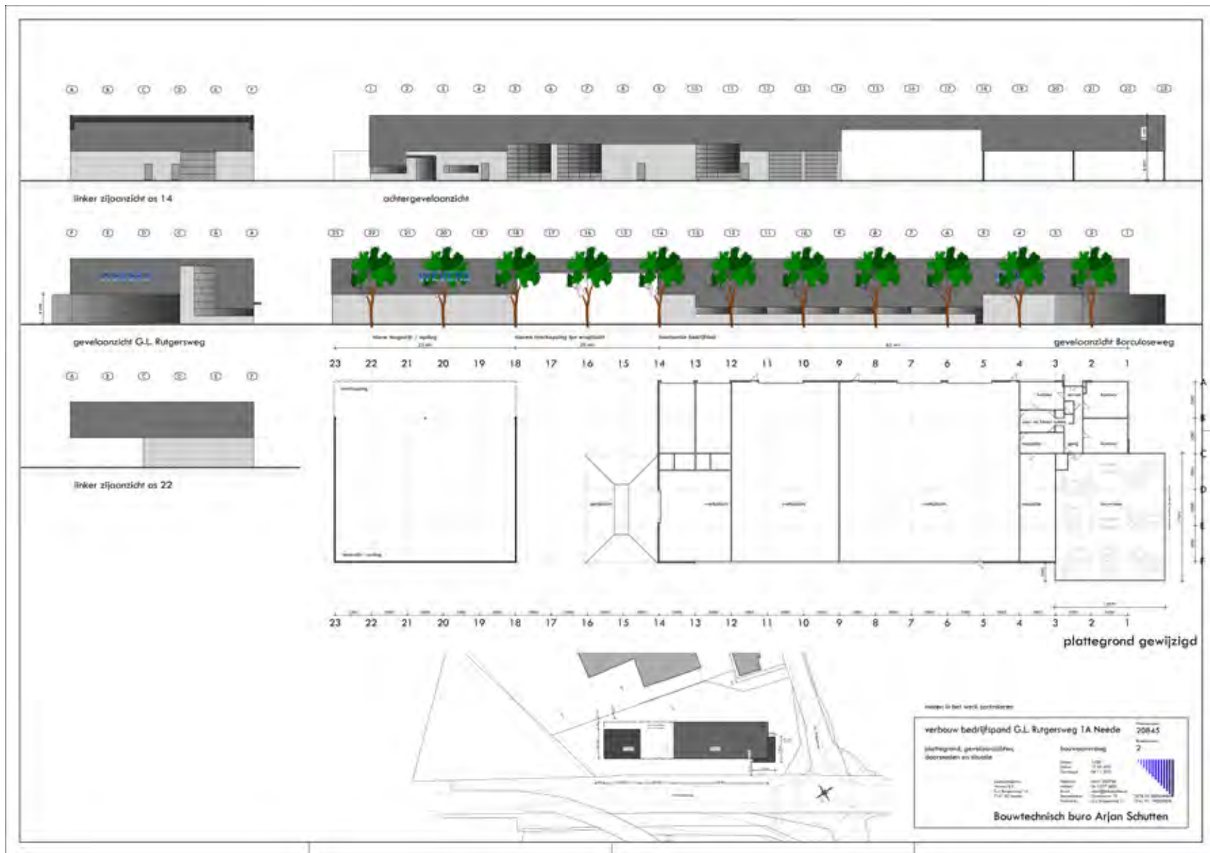
Afbeelding: Plan uitbreiding door Bouwtechnisch bureau Arjan Schutten
