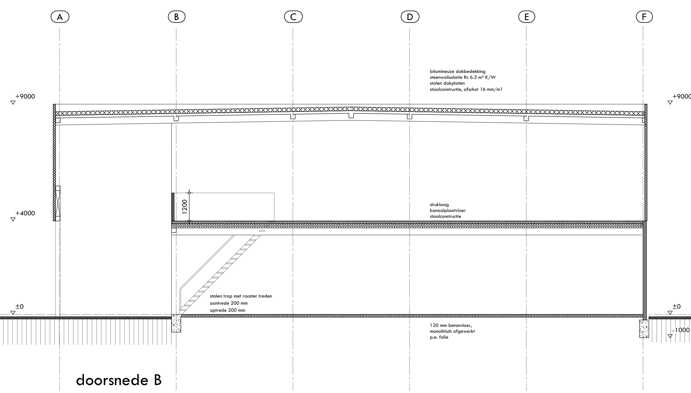
doorsnede B
