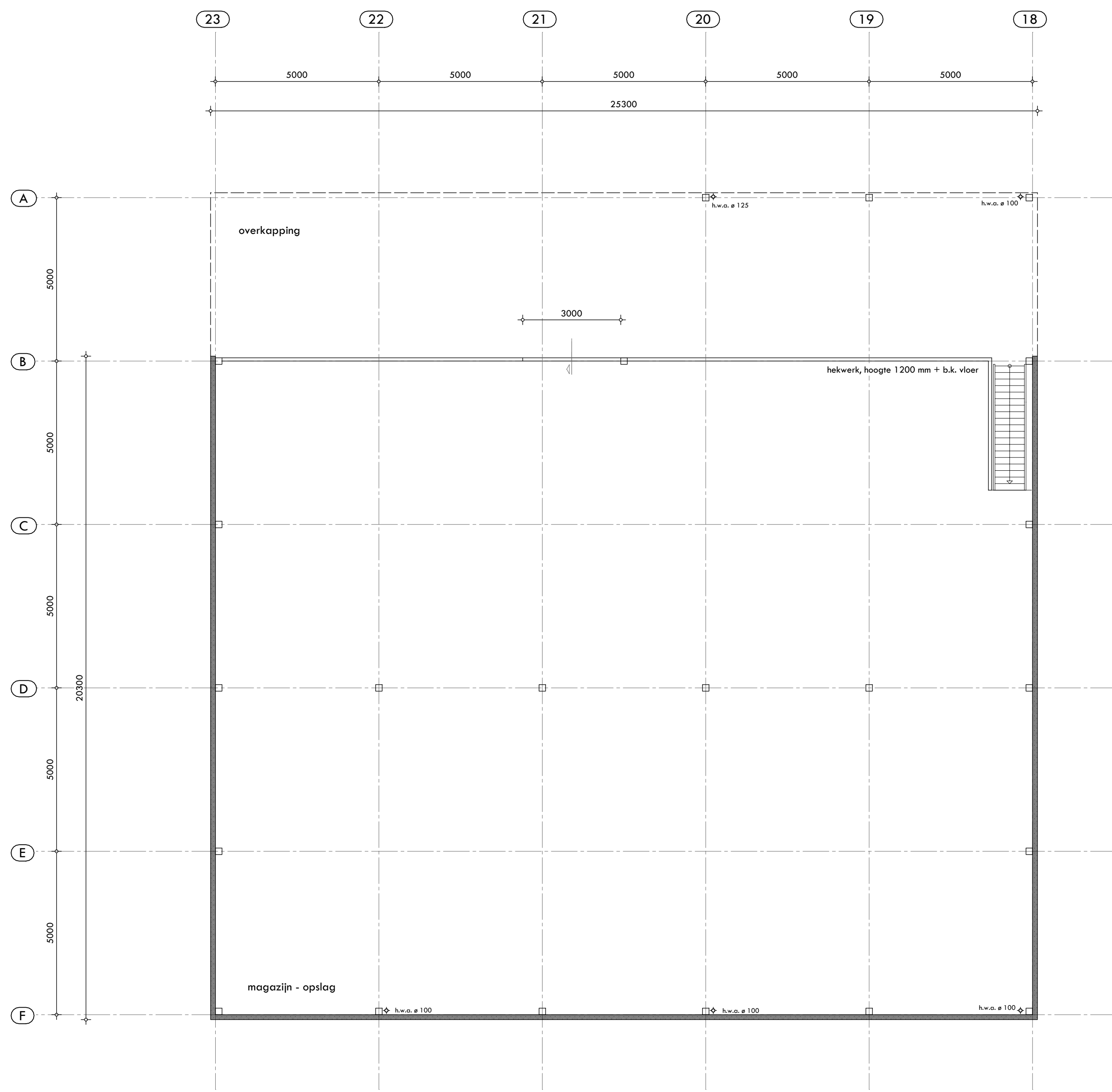
verdieping gewijzigd 4000+
