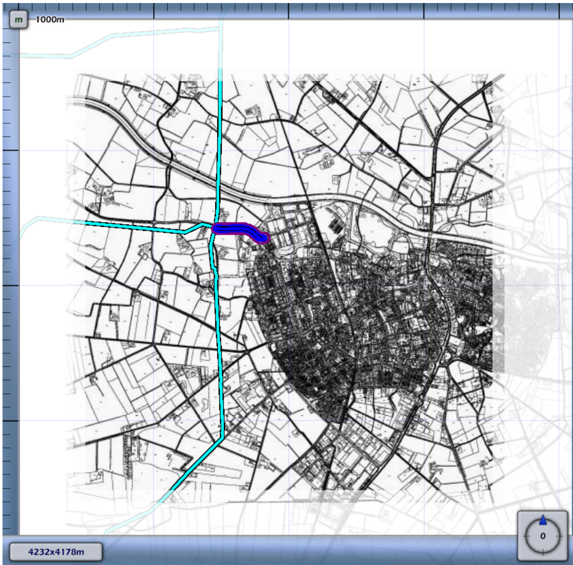
3.1 Figuur 3.1 Plaatsgebonden risico voor N-569-82 van N.V. Nederlandse Gasunie
