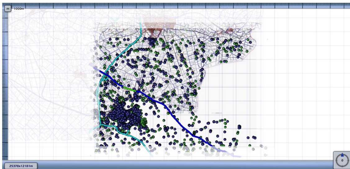
4.4 Figuur 4.4 Groepsrisico screening voor 2081_leiding-N-560-03-deel-1 van N.V. Nederlandse Gasunie
