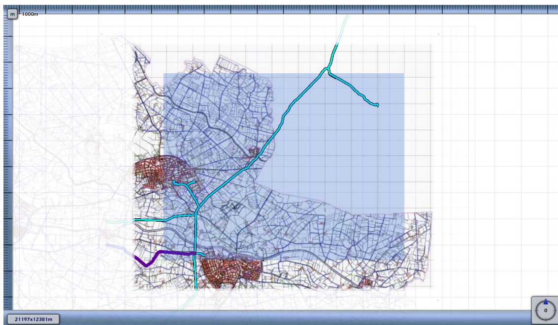
3.8 Figuur 3.8 Plaatsgebonden risico voor 2082_leiding-N-569-81-deel-1_incl verl van N.V. Nederlandse Gasunie
