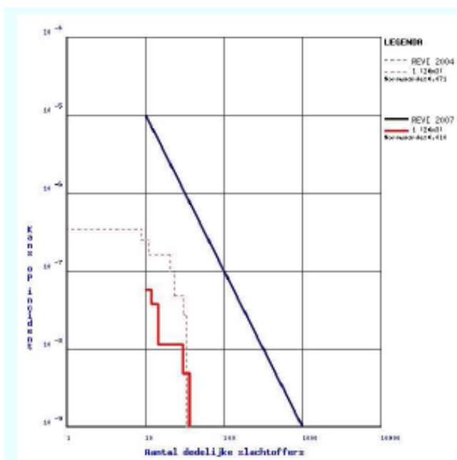
Figuur 10 Groepsrisicocurve Oosterveen's oliehandel BV
