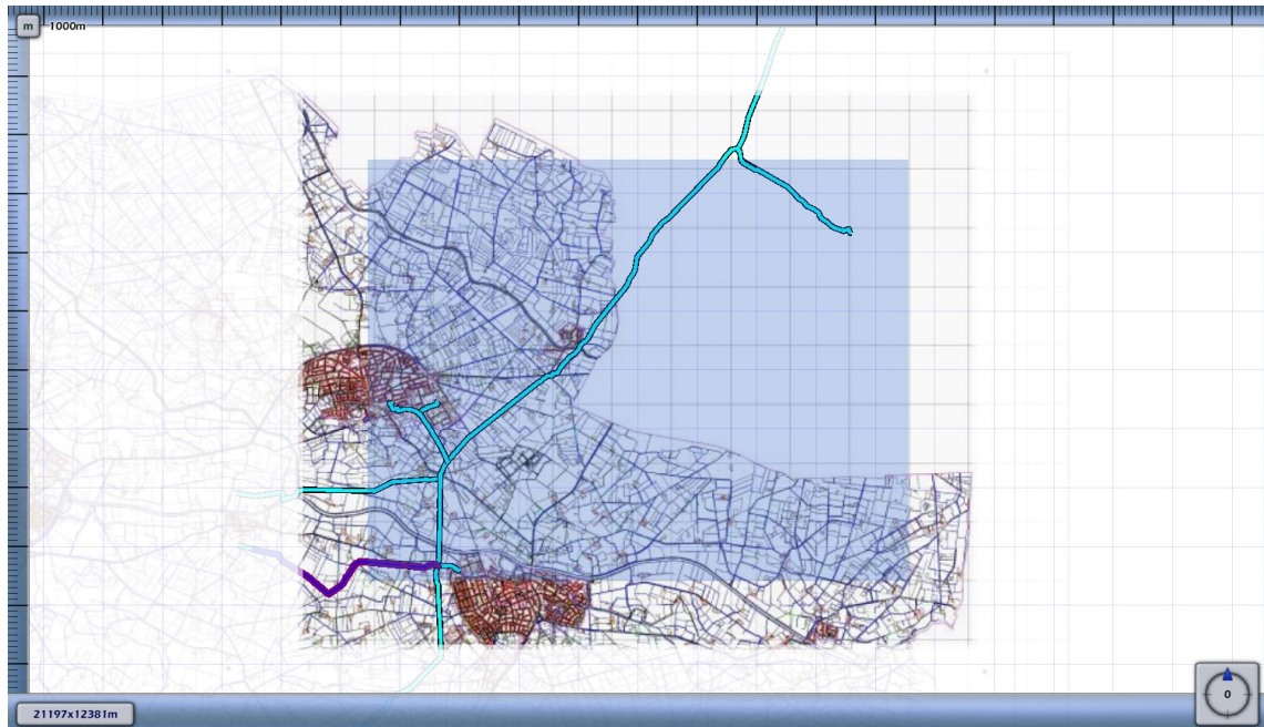
3.10 Figuur 3.10 Plaatsgebonden risico voor 2084_leiding-N-569-80-deel-1_incl verl van N.V. Nederlandse Gasunie
