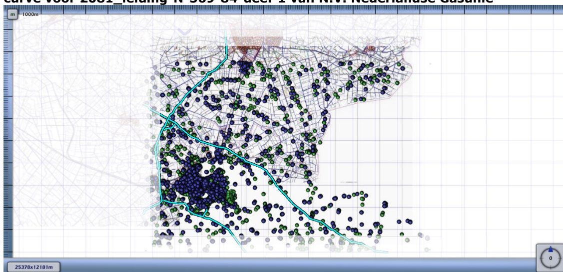
Figuur 4.10 Kilometer leiding behorende bij de maximale overschrijding van de FN-curve voor 2081_leiding-N-569-84-deel-1 van N.V. Nederlandse Gasunie
