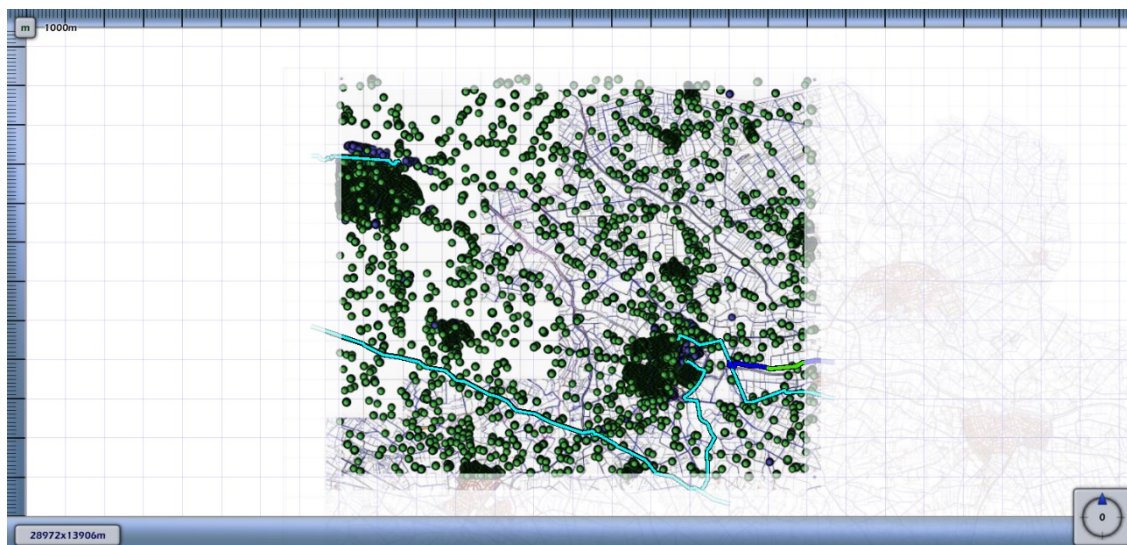
4.10 Figuur 4.10 Groepsrisico screening voor 2078_leiding-N-569-84-deel-1 van N.V. Nederlandse Gasunie
