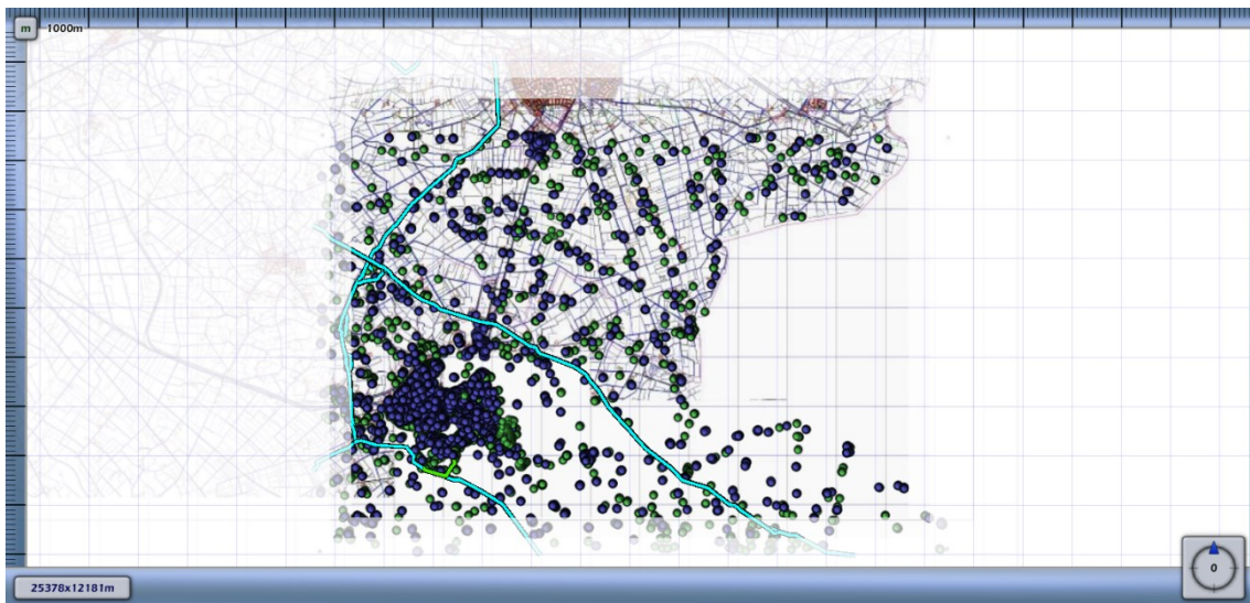
4.7 Figuur 4.7 Groepsrisico screening voor 2081_leiding-N-569-07-deel-1 van N.V. Nederlandse Gasunie
