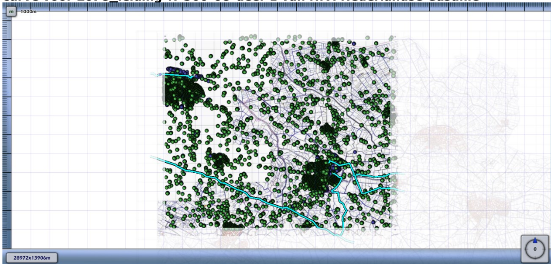
Figuur 4.8 Kilometer leiding behorende bij de maximale overschrijding van de FN-curve voor 2078_leiding-N-560-08-deel-1 van N.V. Nederlandse Gasunie
