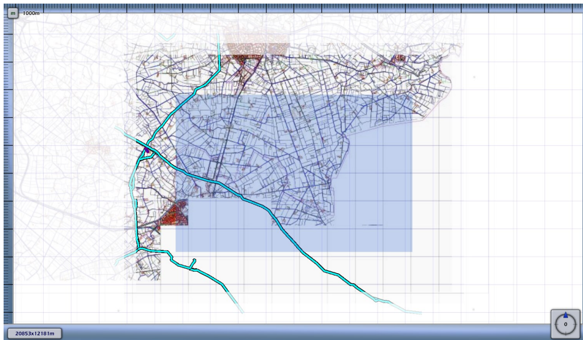
3.8 Figuur 3.8 Plaatsgebonden risico voor 2081_leiding-N-569-79-deel-1 van N.V. Nederlandse Gasunie
