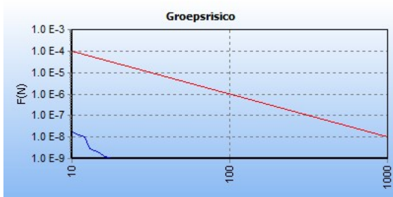
5.4 Figuur 5.4 FN curve voor 2080_leiding-A-628-deel-1 van N.V. Nederlandse Gasunie voor de kilometer tussen stationing 1740.00 en stationing 2740.00
