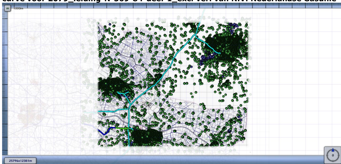
Figuur 4.7 Kilometer leiding behorende bij de maximale overschrijding van de FN-curve voor 2079_leiding-N-569-84-deel-1_excl verl van N.V. Nederlandse Gasunie
