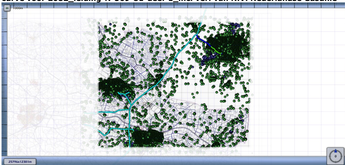
Figuur 4.8 Kilometer leiding behorende bij de maximale overschrijding van de FN-curve voor 2082_leiding-N-569-81-deel-1_incl verl van N.V. Nederlandse Gasunie
