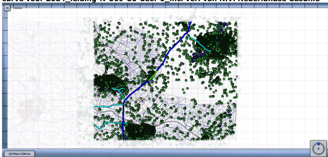
Figuur 4.10 Kilometer leiding behorende bij de maximale overschrijding van de FN-curve voor 2084_leiding-N-569-80-deel-1_incl verl van N.V. Nederlandse Gasunie
