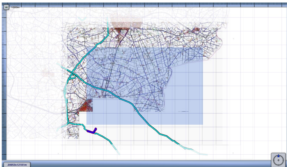
3.12 Figuur 3.12 Plaatsgebonden risico voor 2086_leiding-N-560-06-deel-1_incl verl van N.V. Nederlandse Gasunie
