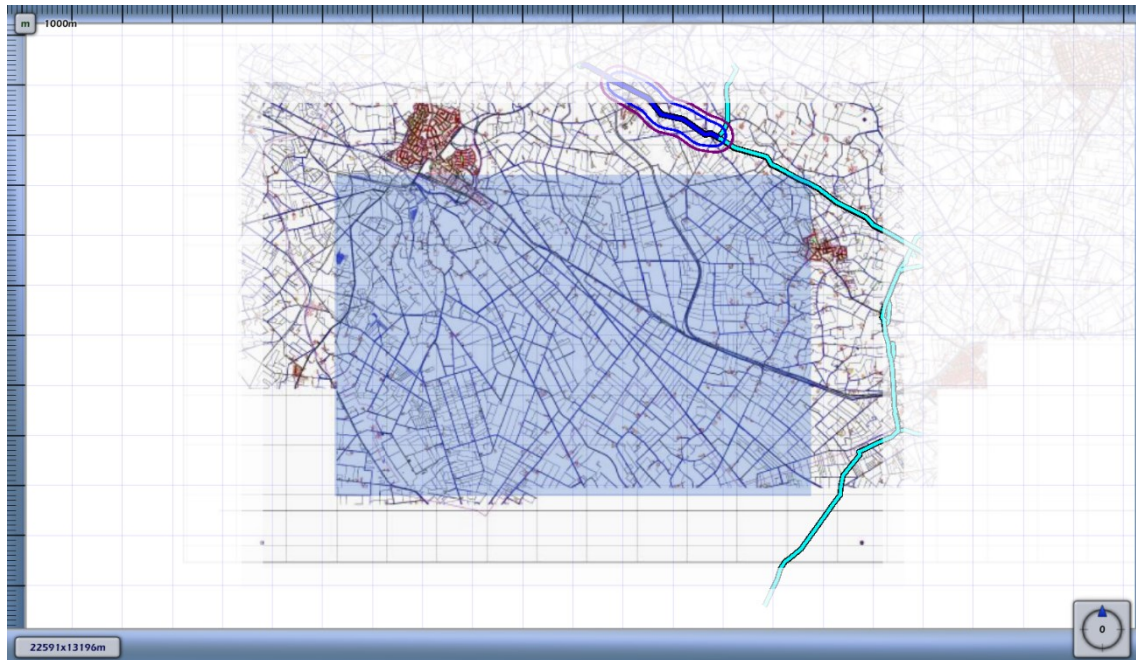
3.6 Figuur 3.6 Plaatsgebonden risico voor 2080_leiding-N-560-03-deel-1 van N.V. Nederlandse Gasunie
