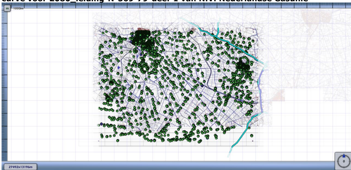
Figuur 4.8 Kilometer leiding behorende bij de maximale overschrijding van de FN-curve voor 2080_leiding-N-569-79-deel-1 van N.V. Nederlandse Gasunie
