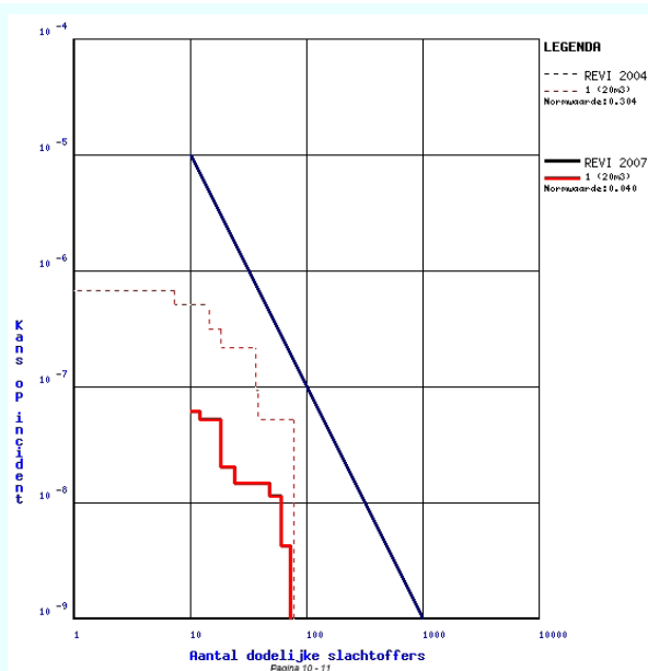
Figuur 6 FN curve Kanter's motorbrandstoffen Ruurlo
