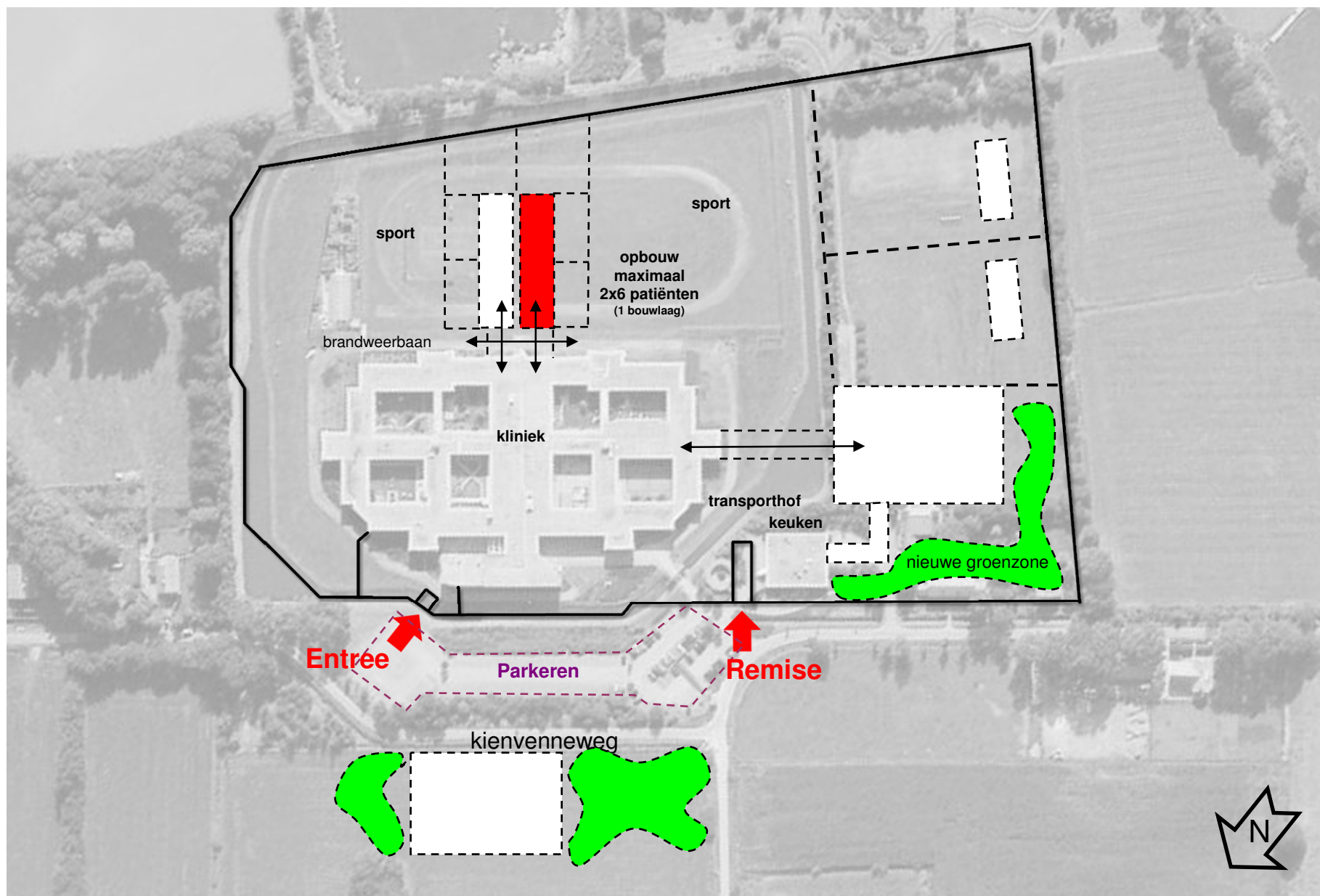
FPC Oldenkotte Rekken, Vervanging 2x6 patiënten fase 3
