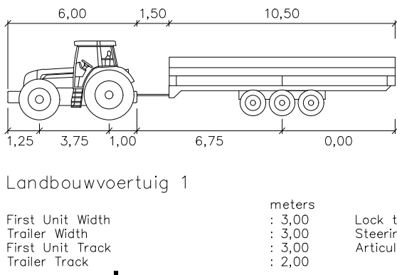
Rijcurve landbouwvoertuig vanuit Molenlaan SCHAAL 1 : 500
