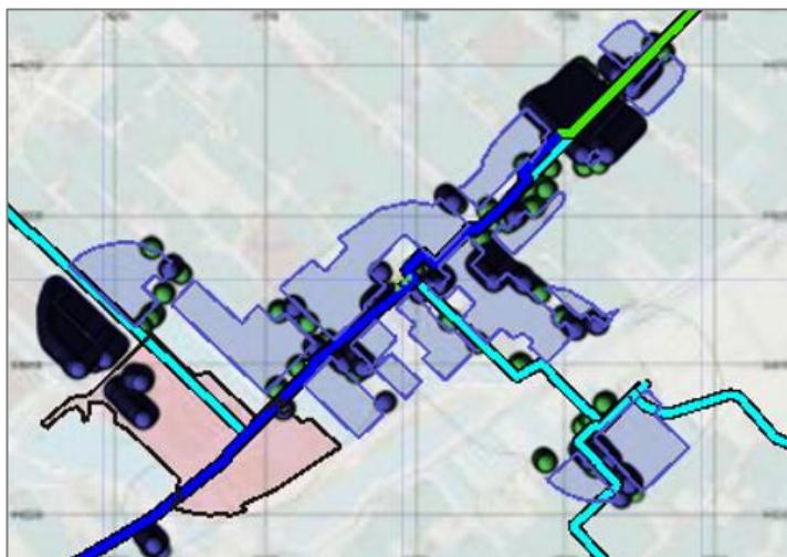
Figuur 5. W-509-01: — kilometer leiding met het hoogste GR
