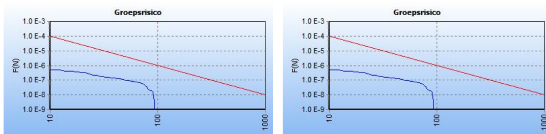
Figuur 3. Groepsrisico W-509-01, huidig (links) en toekomstig (rechts)
