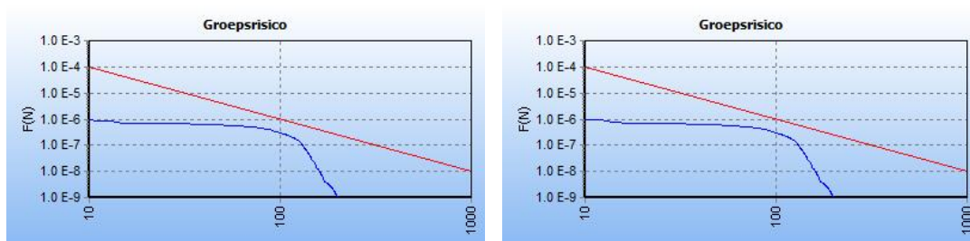
Figuur 4. Groepsrisico W-522-01, huidig (links) en toekomstig (rechts)
