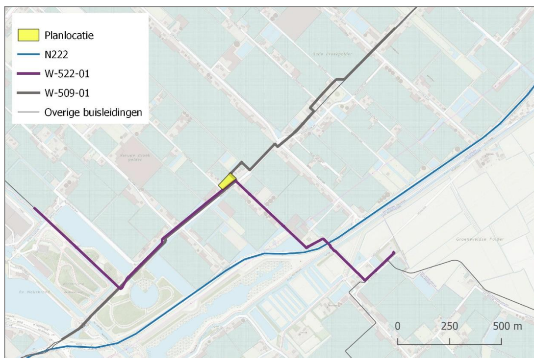
Figuur 1. Plangebied, hogedruk aardgasleidingen en N222
