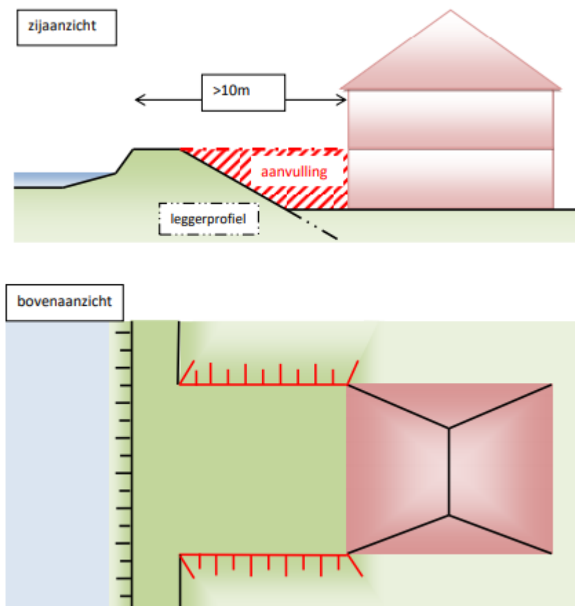
Figuur 3.3: Bouwafstand bij aanhelen en Bouwafstand bij aanvullen op kruinhoogte (Bron: Beleidsregel Medegebruik waterkeringen, Delfland)
