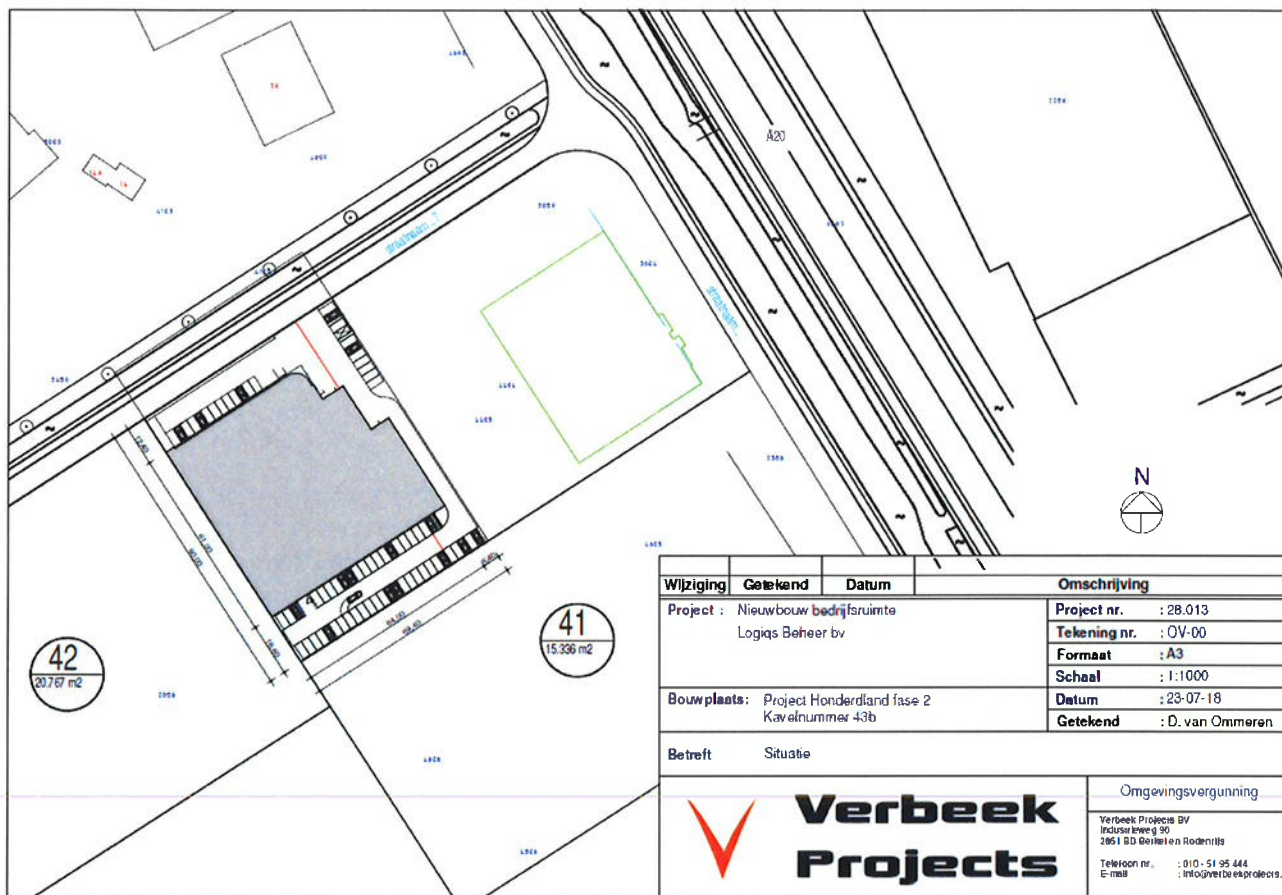
Figuur 2: Situatietekening van Logiqs op een gedeelte van AGE 43, zijnde AGE 43b.
