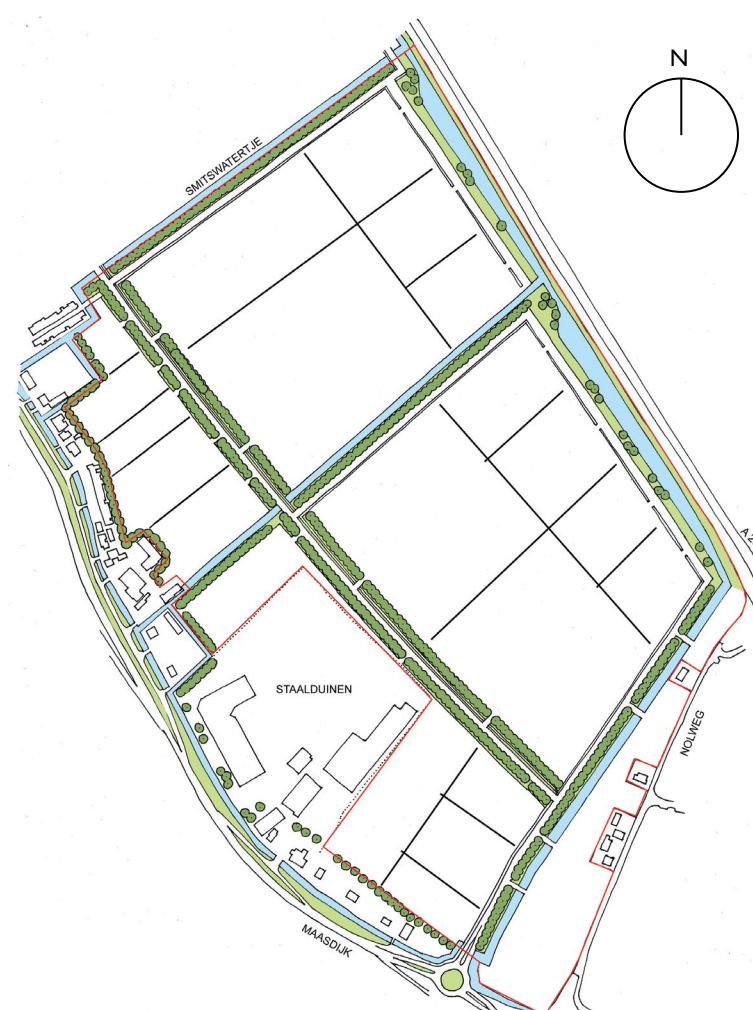
Masterplan fase I, met de plangrens aangegeven
