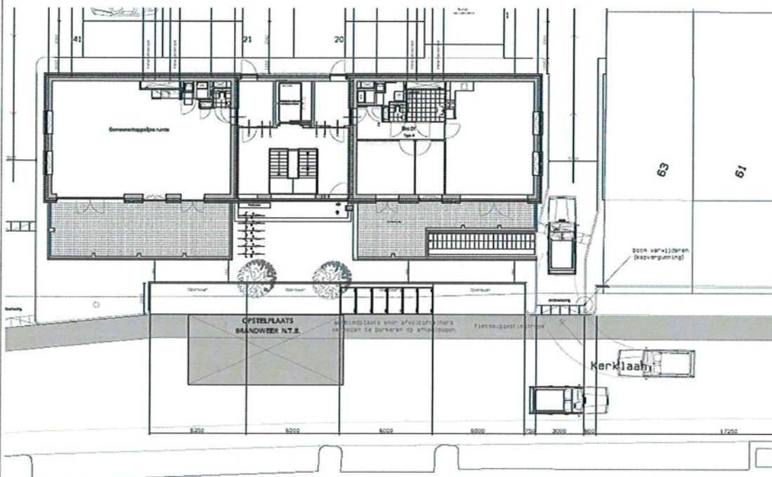
Aangepaste situatietekening.
