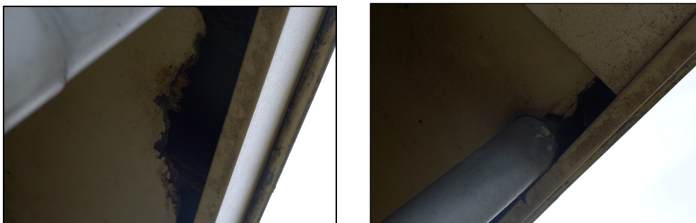
Figuur 3.2.3: Gaten in de houten dakrandconstructie die toegang voor vleermuizen bieden tot de dakconstructie en/of de spouwmuur van de woning.
