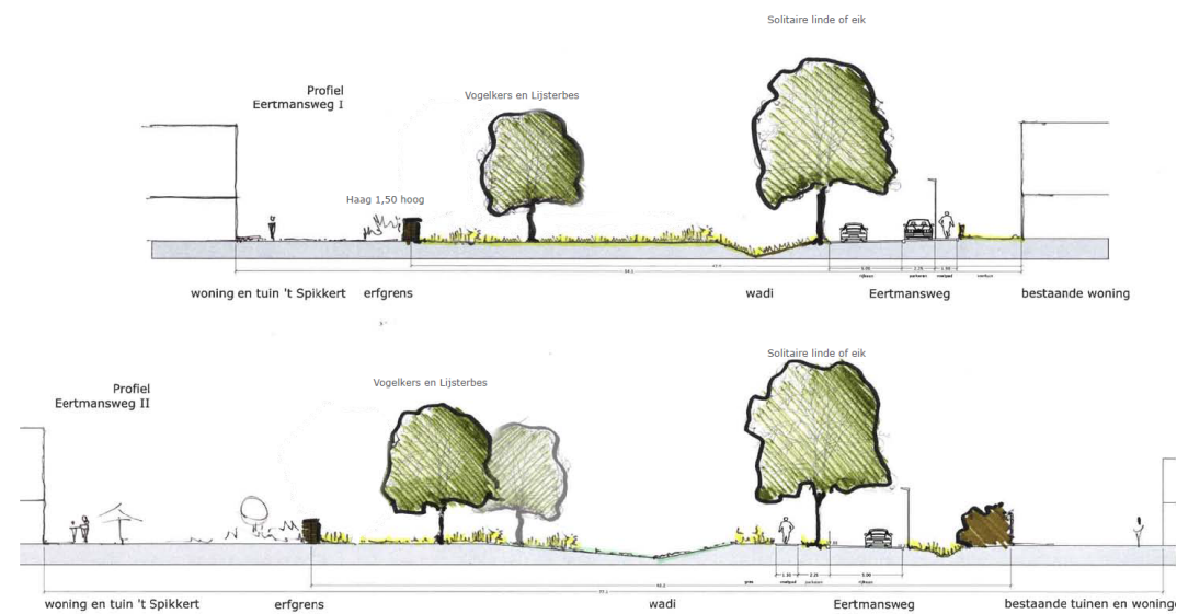
Principedoorsnede Eertmansweg
