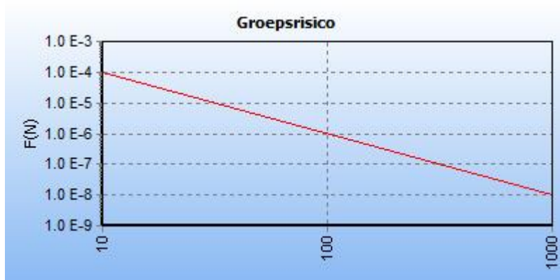
Figuur 5.1 FN curve bestaande situatie voor 7981_leiding-N-531-91-deel-1 van N.V. Nederlandse Gasunie voor de kilometer tussen stationing 1150.00 en stationing 2150.00
