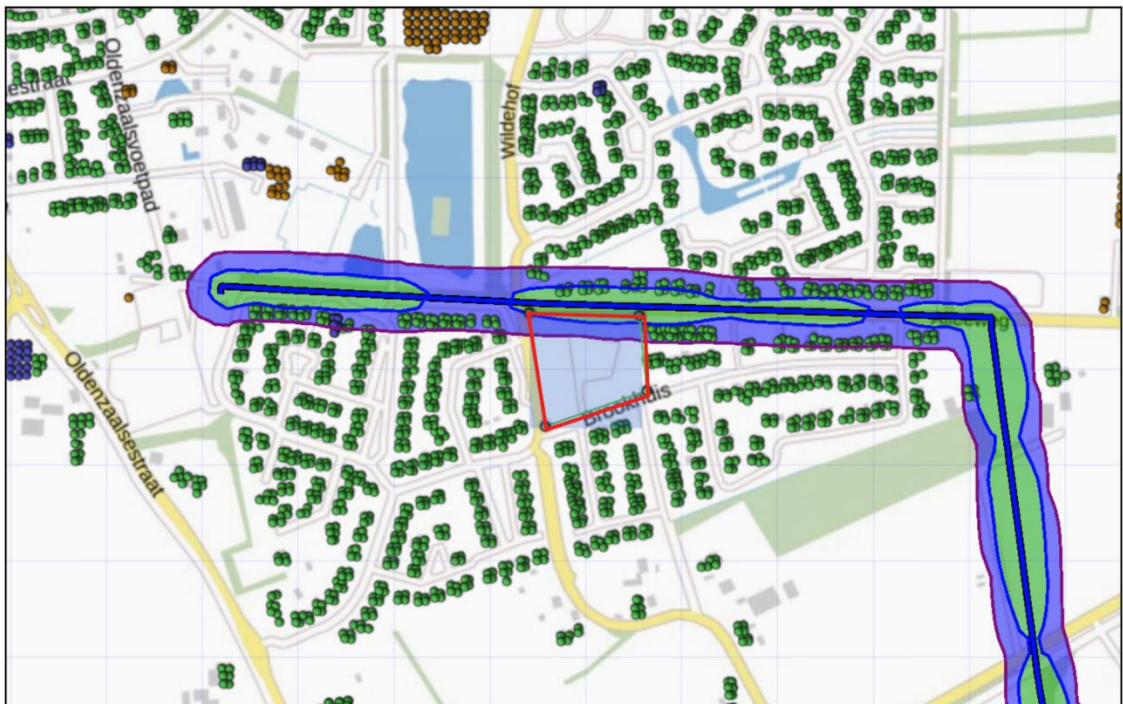
Figuur 3.1 Plaatsgebonden risico voor 7177_leiding-N-531-91-deel-1 van N.V. Nederlandse Gasunie
