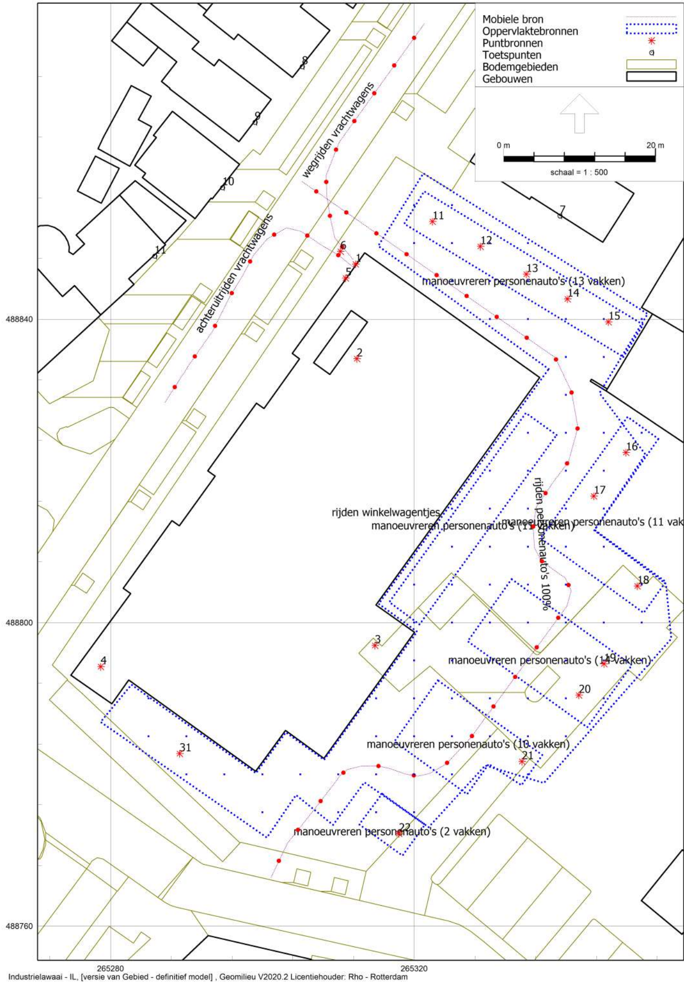
Bijlage 2.2: overzicht van het akoestisch rekenmodel met de ligging van de geluidbronnen
