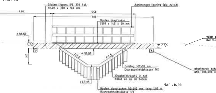
Zijaanzicht nieuwe brug op basis van profiel D - D'
