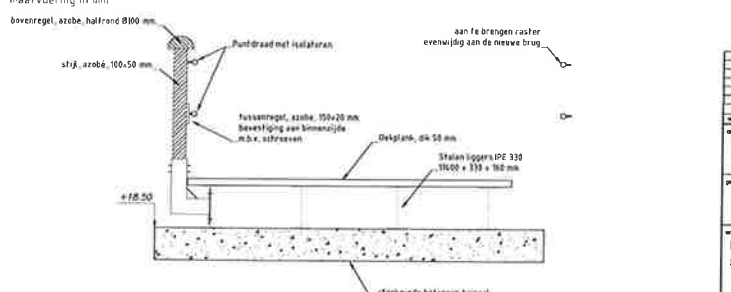
Doorsnede over de as schaal 1:20 maatvoering in mm
