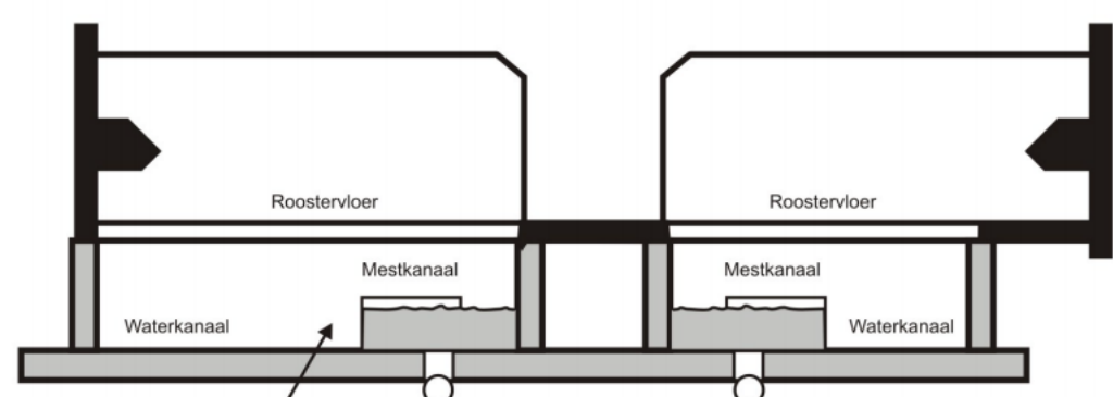
Detail stalsysteem BWL 2004.07.V1
