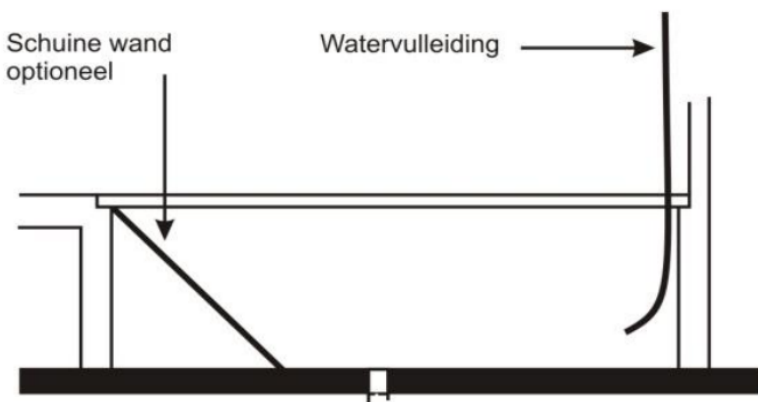
Detail stalsysteem BWL 2006.07.V2
