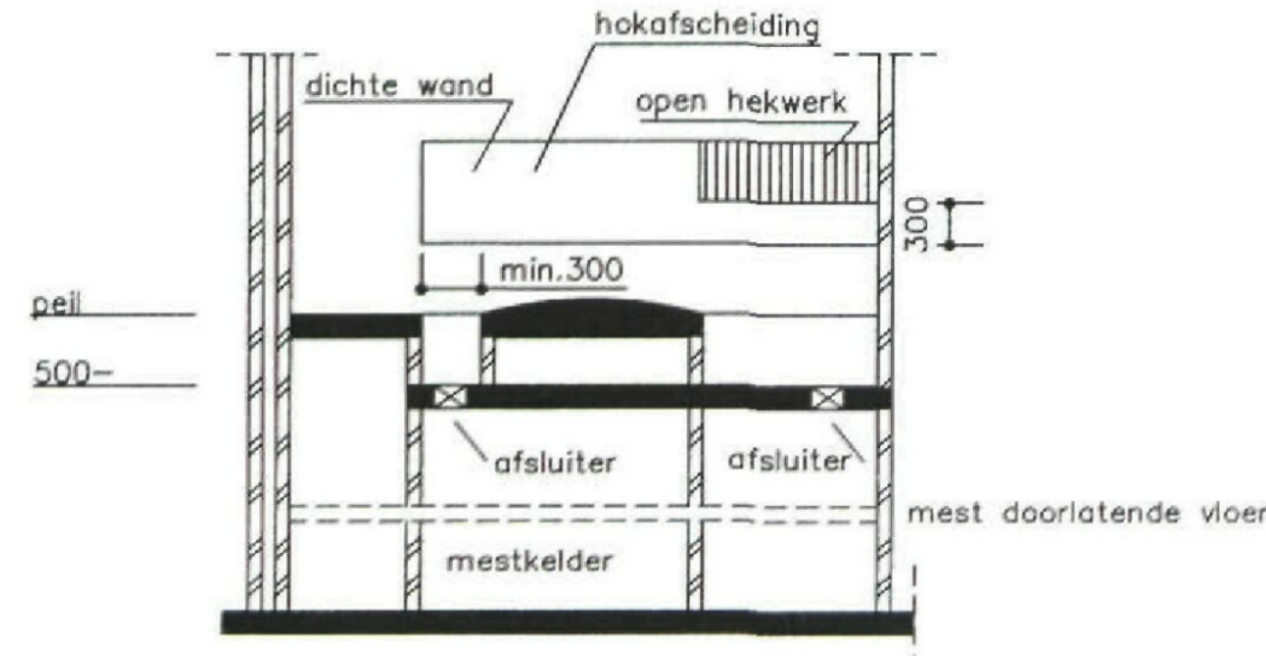
Detail stalsysteem BB 96.03.033V2
