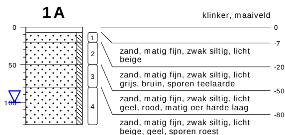
type grondboring datum 15-03-2017 boormeester Jan Hartman
