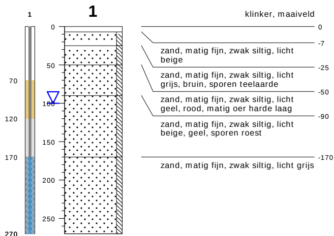
type peilbuis met 1 filter datum 08-03-2017 boormeester Jan Hartman
