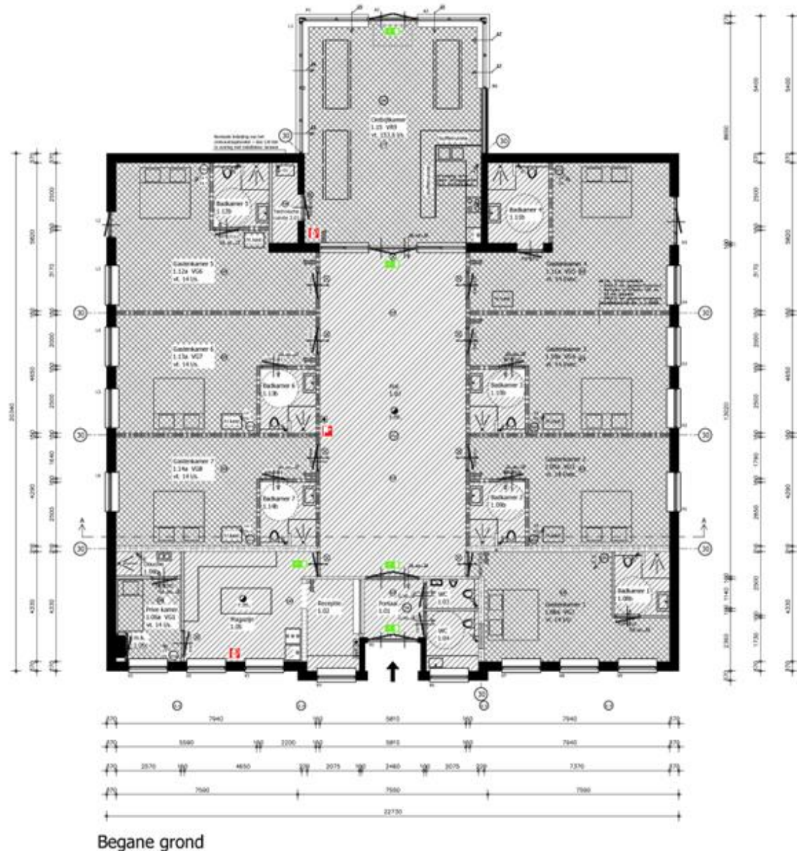
Afbeelding 2.4: gewijzigde plattegrond begane grond
