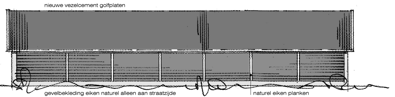
zijgevels
