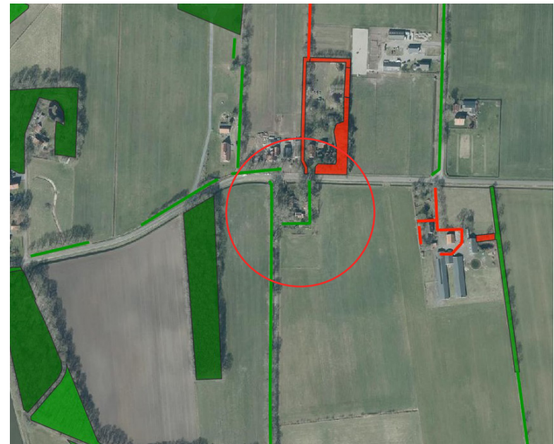
Fragmenten van de cascokaart behorende bij de casco benadering. Boven: Westelhoekweg 10. Onder: Punthuizerweg 30. (Bron: geo.overijssel.nl )
