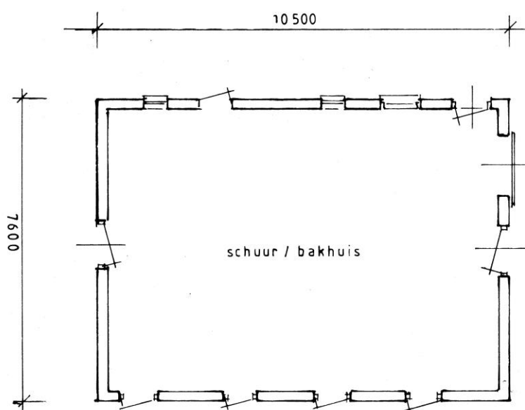
Plattegrond
